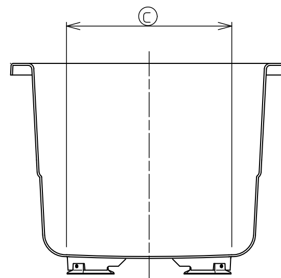
A-A断面(最も広い位置)
