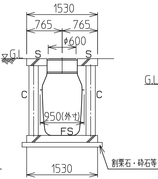
B-B'断面図
