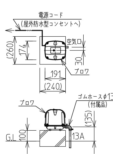
プロフ据付図(例) (尺度 N.T.S.)
