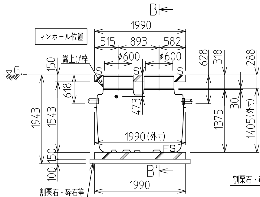
A-A'断面図
