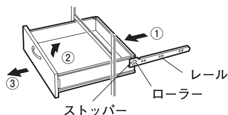
<取外し方法>
