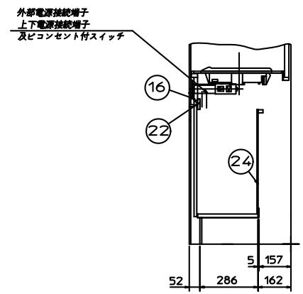
断面CC
