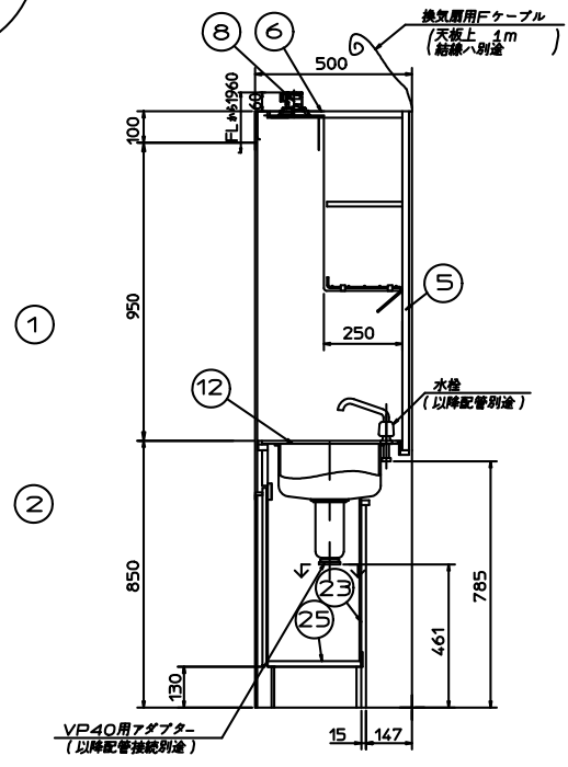
断面BB
