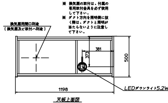
天板上面図
