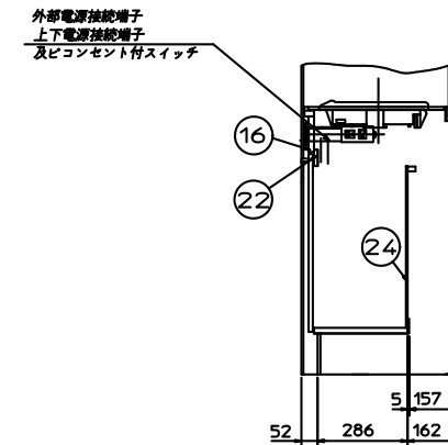
断面CC
