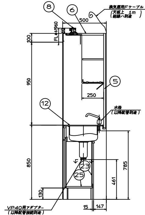
断面BB
