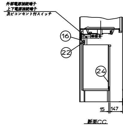
断面CC
