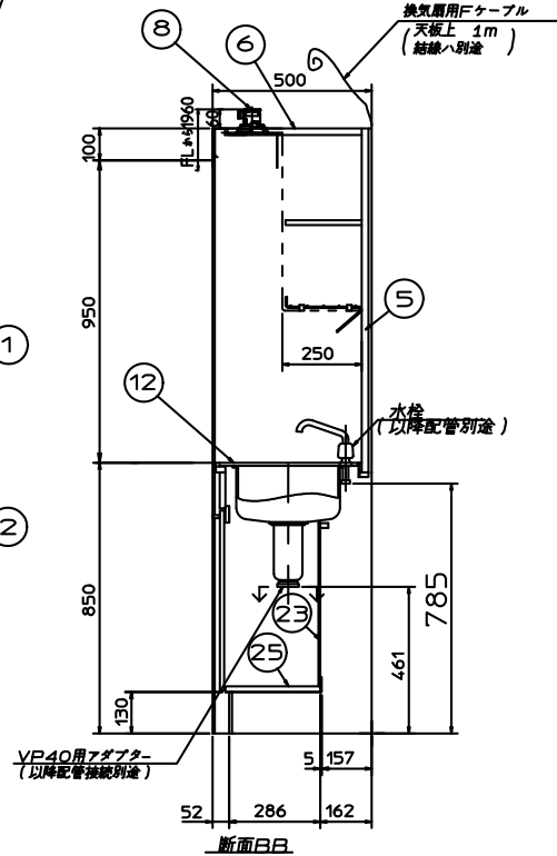
断面BB
