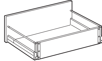
B タイプ (プルモーション機能あり) 最大積載量：20 kg (中段引出しのみ 35kg)
