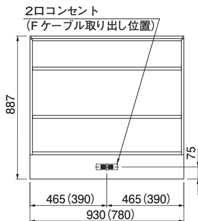
正面図
