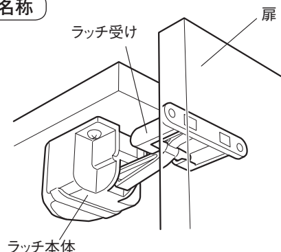
各部の名称
