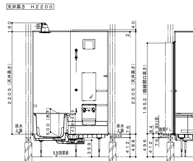
1階設置・ボルト脚
