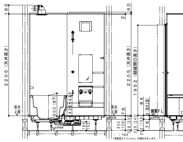
階上設置・ボルト脚
