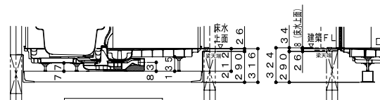
階上設置・吊り架台
