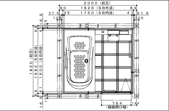
平面図
