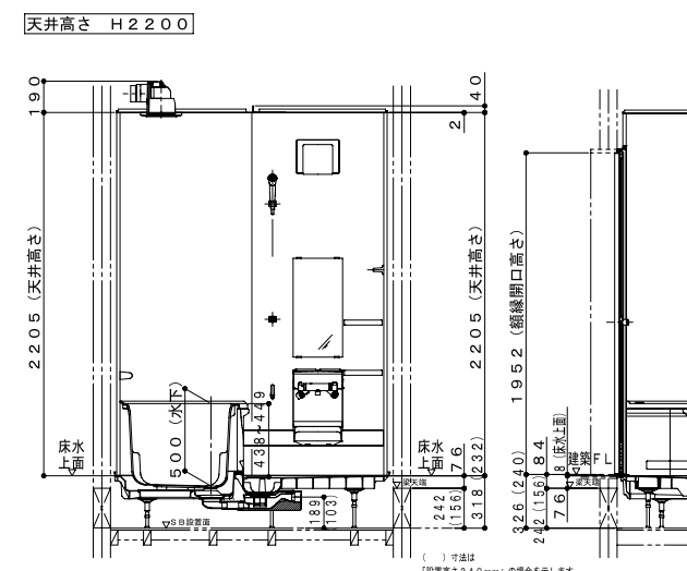
階上設置・ボルト脚
