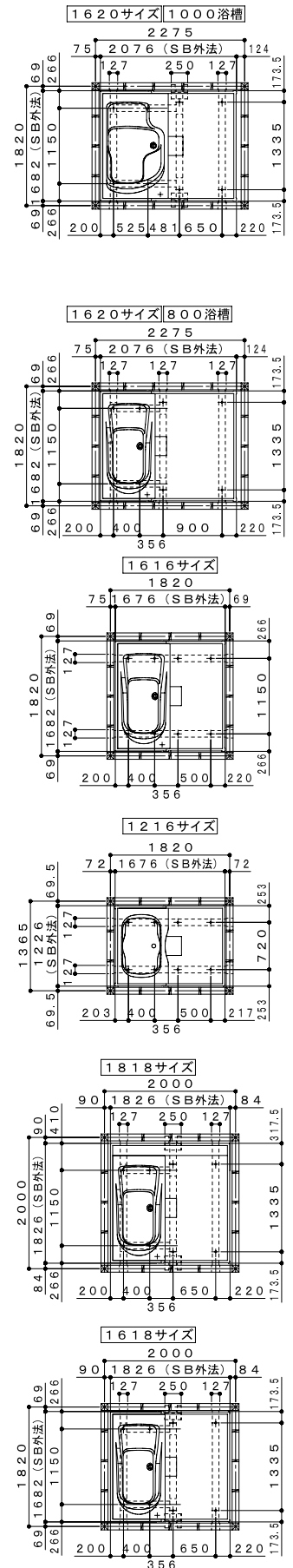
吊り架台位置図
