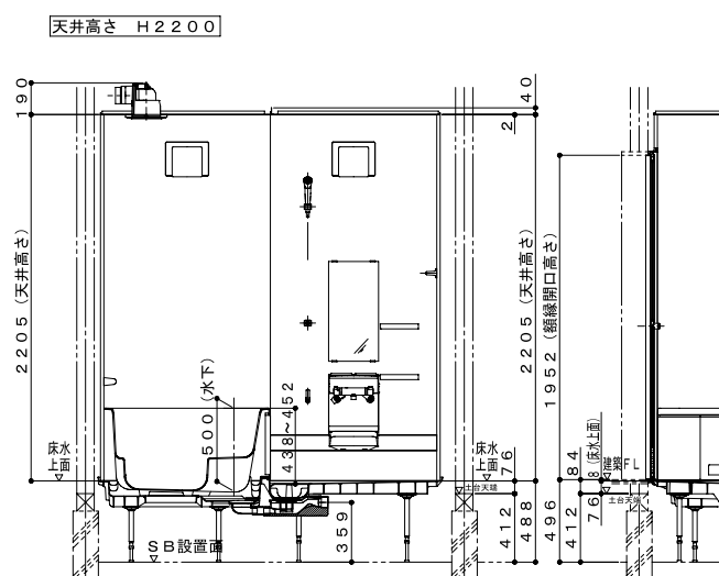
1 階設置・ボルト脚
