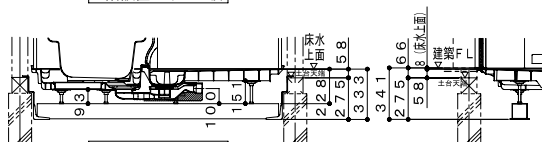
1階設置・吊り架台
