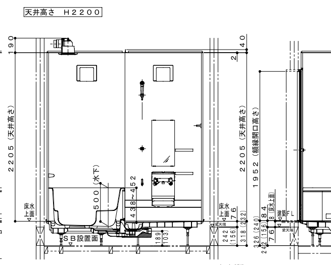
階上設置・ボルト脚
