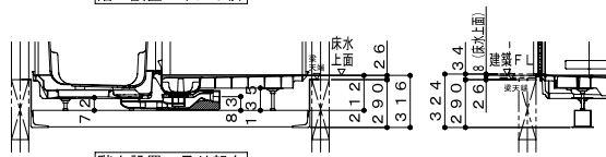
階上設置・吊り架台
