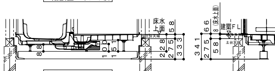
1階設置・吊り架台
