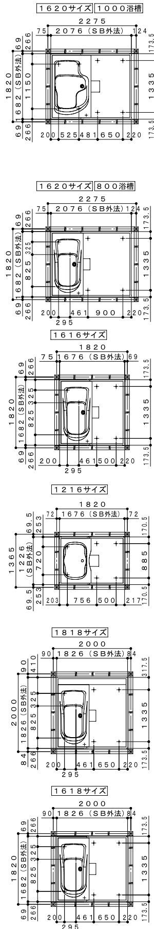
ボルト脚位置図
