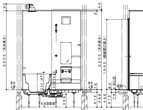
1階設置・ボルト脚
