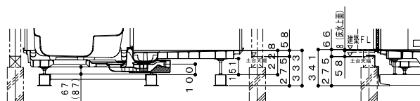
1 階設置・吊り架台
