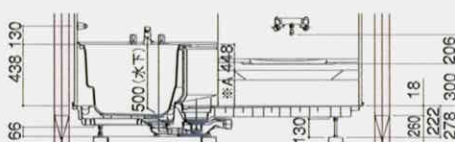
＜階上設置吊り架台仕様＞
