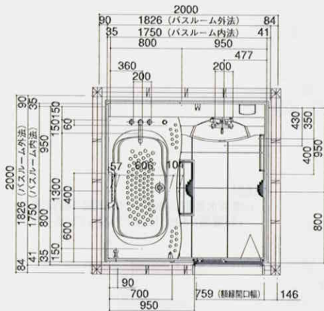
Aセット:セミロングプラン
