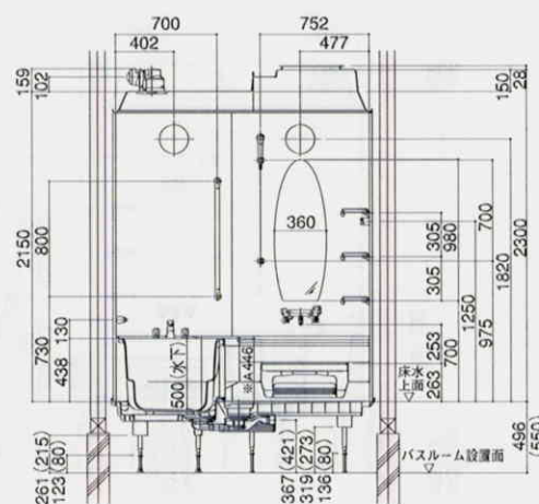
nセット:軟水ピッチ専用セミロングプラン
