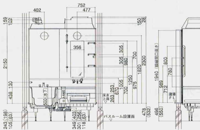
〈1階設置ボルト脚仕様〉
