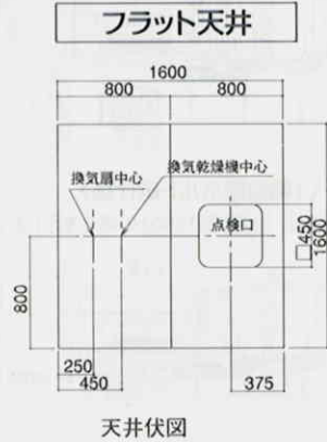
天井伏図
