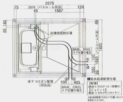
給水給湯配管取出位置図 (配管あり、銅管仕様の場合)
