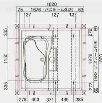
吊り架台位置図
