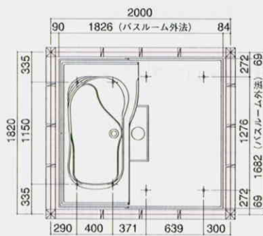
ボルト脚位置図
