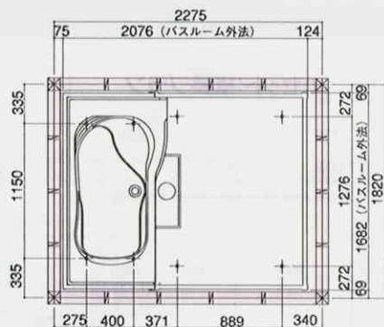
ボルト脚位置図
