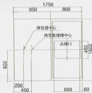
天井伏図
