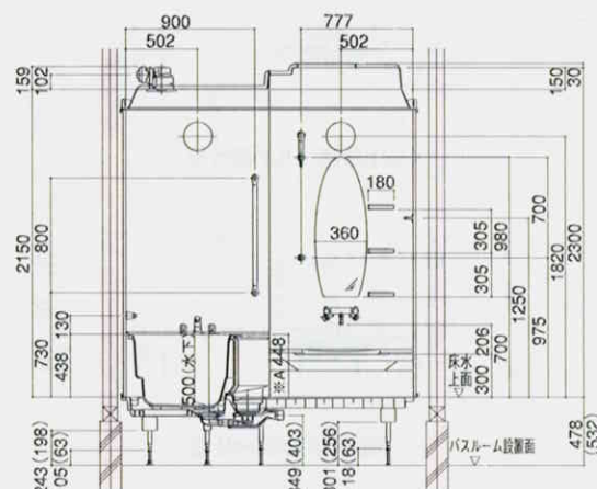
Dセット:オーバル形プラン
