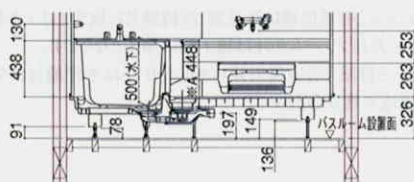
〈階上設置ボルト脚仕様〉
