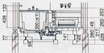
〈1階設置吊り架台仕様〉
