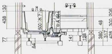
〈1階設置吊り架台仕様〉
