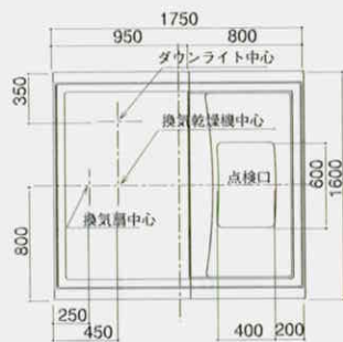
天井伏図
