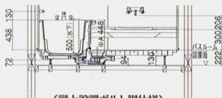
〈階上設置ボルト脚仕様〉
