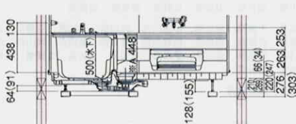
〈階上設置吊り架台仕様〉
