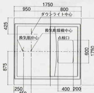
天井伏図
