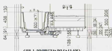
〈階上設置吊り架台仕様〉
