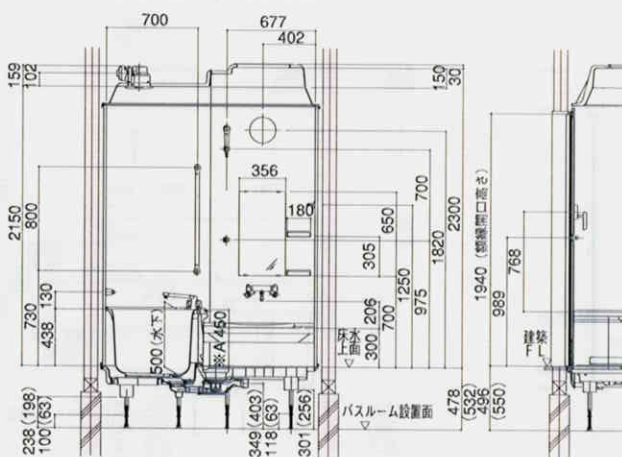
〈1階設置ボルト脚仕様〉
