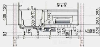
〈階上設置ボルト脚仕様〉
