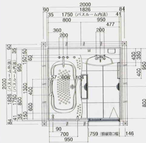
Aセット:セミロングプラン
