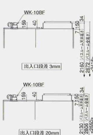
天井断面図
