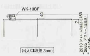
天井断面図
