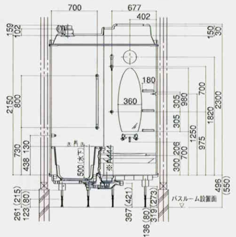
Dセット:オーバル形プラン
