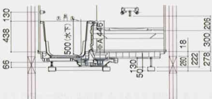
〈階上設置吊り架台仕様〉
