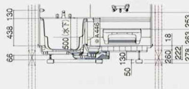
〈階上設置吊り架台仕様〉
