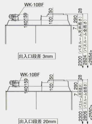
天井断面図
