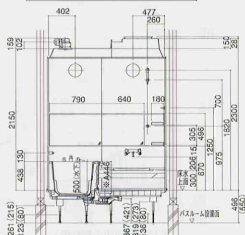
Cセット:横長プラン
