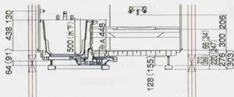
〈階上設置吊り架台仕様〉
