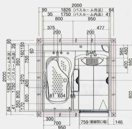
bセット:ロングプラン
