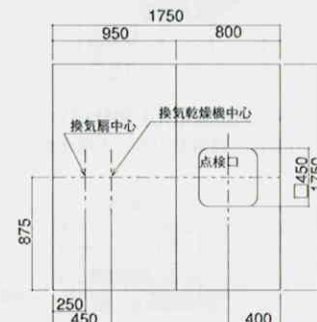
天井伏図
