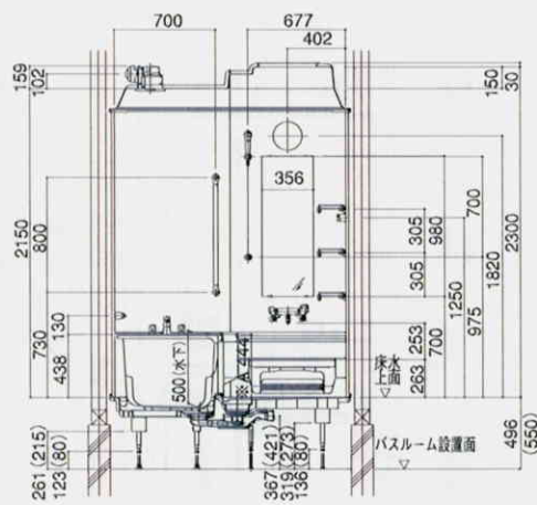
&lt;1階設置ボルト脚仕様&gt;
