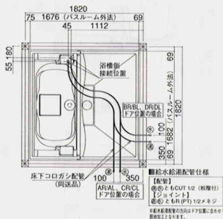
給水給湯配管取出位置図 (配管あり、銅管仕様の場合)
