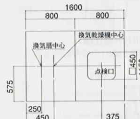
天井伏図
