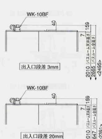
天井断面区
