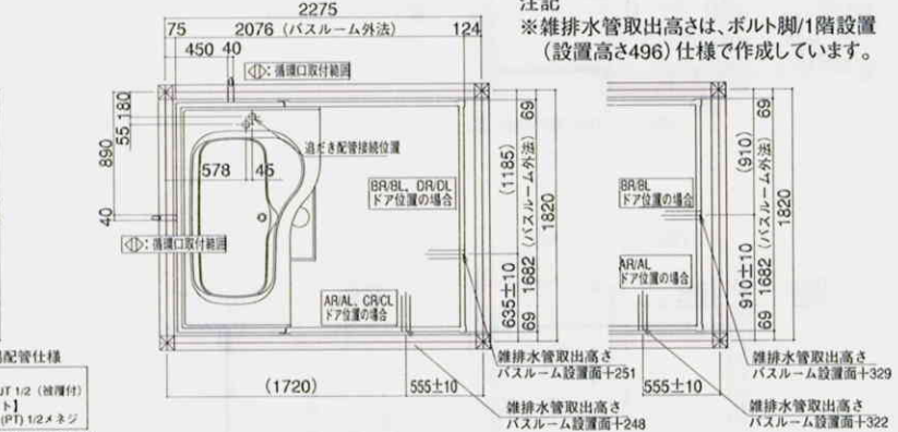
雄排水管取出推奨位置図 循環口取付範囲図
