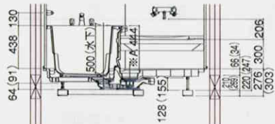
＜階上設置吊り架台仕様＞
