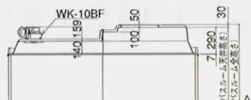
出入口段差 20mm
