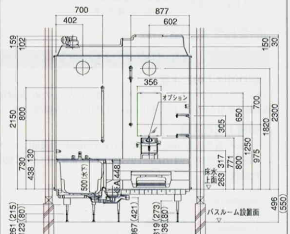
nセット:軟水ピッチ専用セミロングプラン
