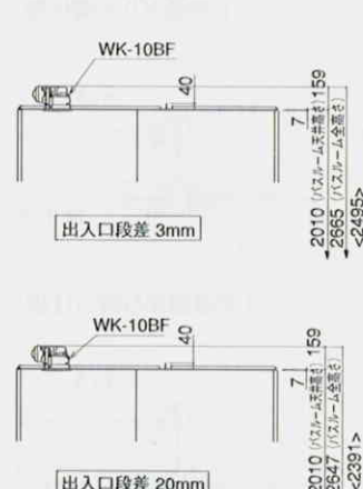
天井断面図
