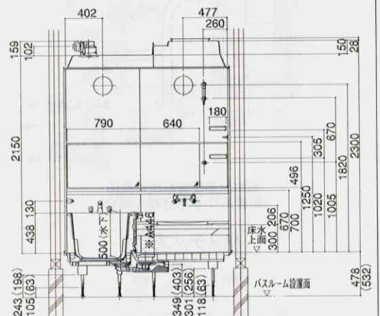
Cセット:横長プラン
