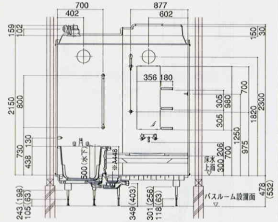
Cセット:横長プラン
