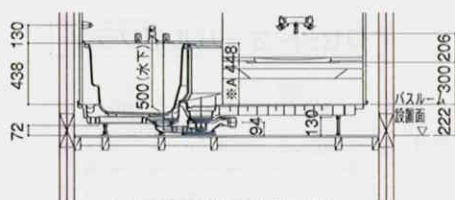
＜階上設置ボルト脚仕様＞
