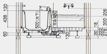
〈階上設置吊り架台仕様〉
