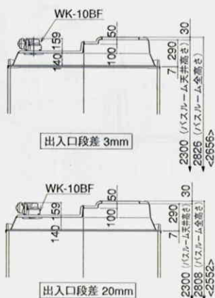
天井断面図
