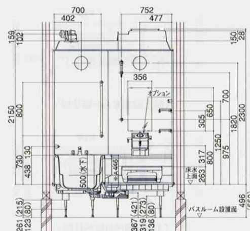
nセット:軟水ピッチ専用セミロングプラン
