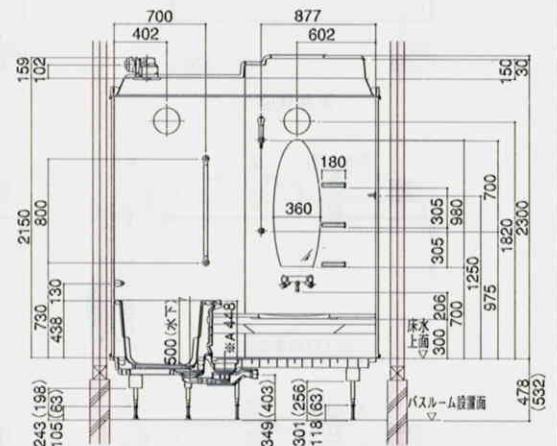
Dセット:オーバル形プラン
