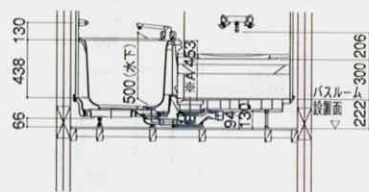
〈階上設置ボルト脚仕様〉
