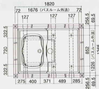
吊り架台位置図
