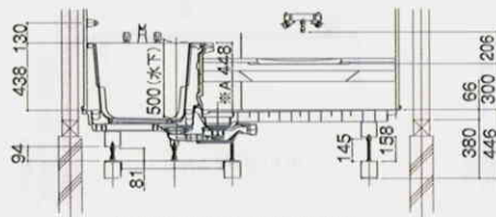
〈1階設置吊り架台仕様〉
