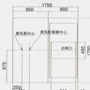
天井伏図
