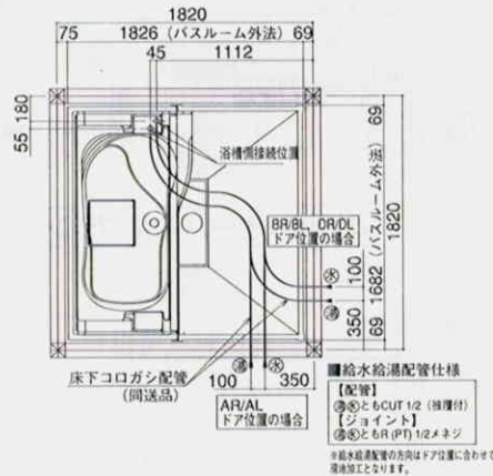
給水給湯配管取出位置図 (配管あり、銅管仕様の場合)
