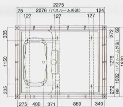
吊り架台位置図
