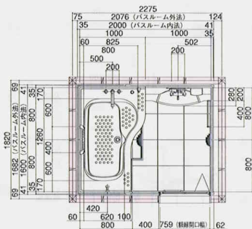
Aセット:セミロングプラン
