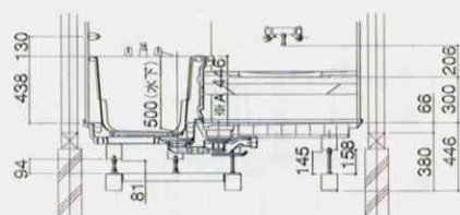
〈1階設置吊り架台仕様〉
