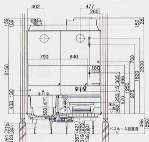
dセット:オーバル形プラン
