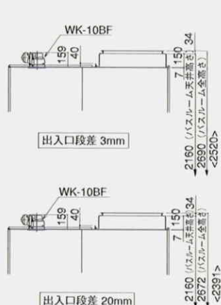
天井断面図
