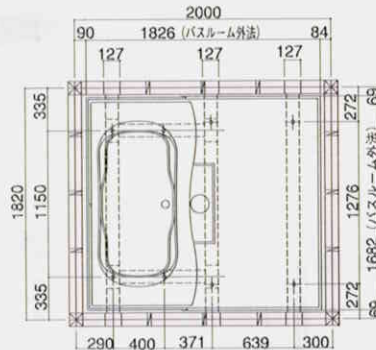
吊り架台位置図
