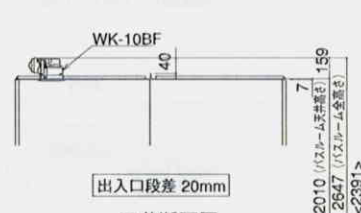
天井断面図
