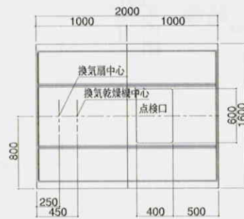
天井伏図
