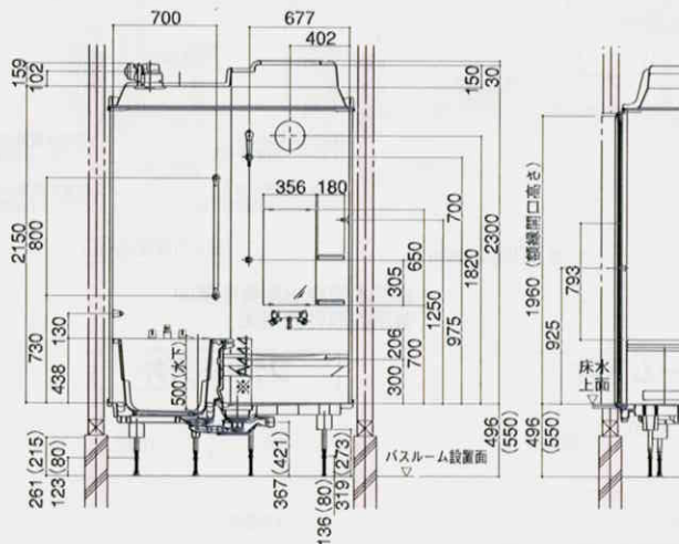
＜1階設置ボルト脚仕様＞
