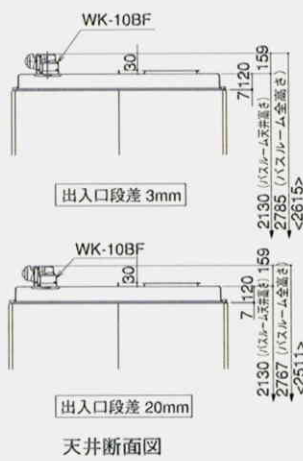
天井断面図
