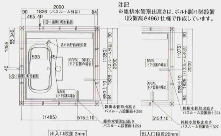
給排水管取出推奨位置図 循環口取付範囲図
