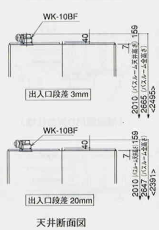
天井断面図
