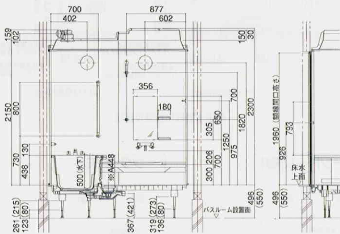
＜1階設置ボルト脚仕様＞
