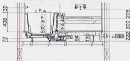
〈階上設置ボルト脚仕様〉
