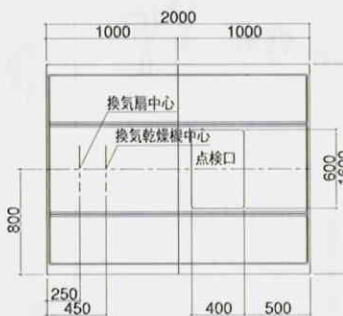
天井伏図
