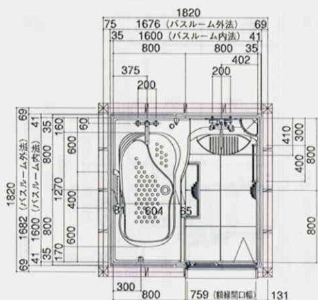
bセット:ロングプラン
