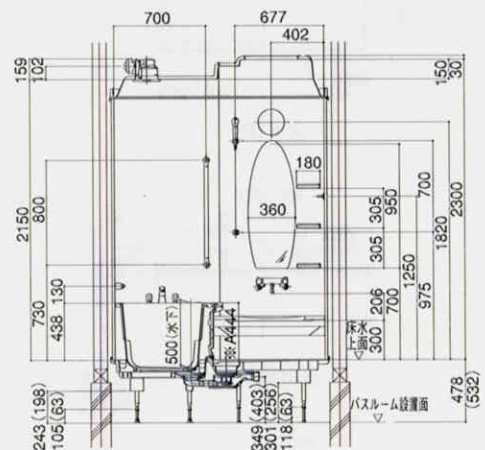
Dセット:オーバル形プラン
