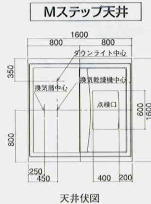
天井伏図
