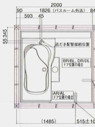
吊り架台位置図
