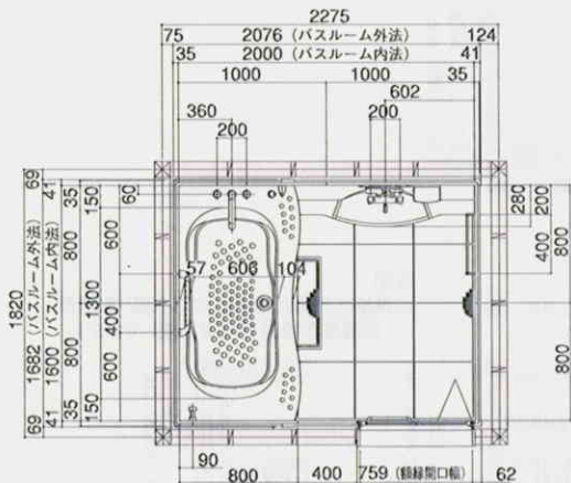
Aセット:セミロングプラン
