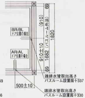
出入口段差 20mm
