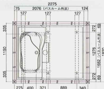
吊り架台位置図
