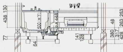
〈1階設置吊り架台仕様〉
