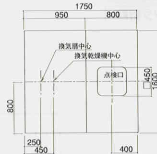
天井伏図
