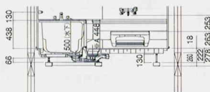
〈階上設置吊り架台仕様〉
