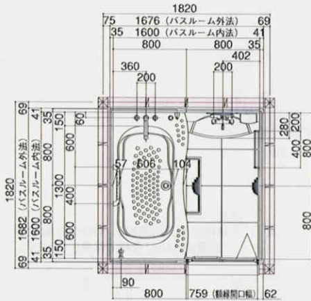
Aセット:セミロングプラン
