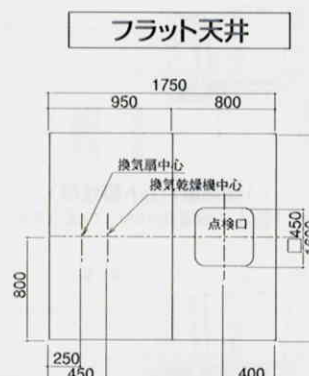
天井伏図
