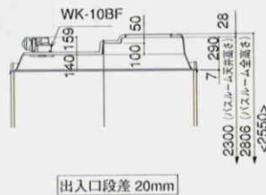
天井断面図
