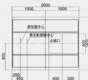
天井伏図
