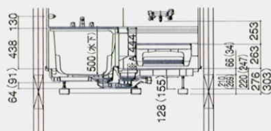
&lt;階上設置吊り架台仕様&gt;
