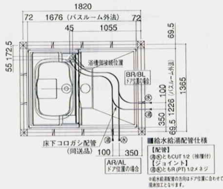
給水給湯配管取出位置図 (配管あり、銅管仕様の場合)
