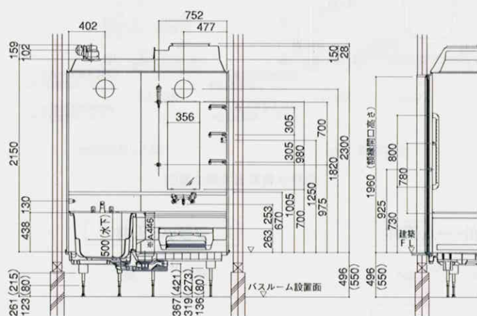
〈1階設置ボルト脚仕様〉
