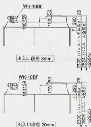
天井断面図
