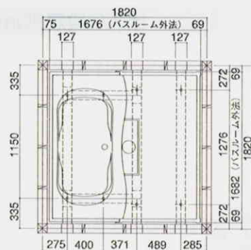
吊り架台位置図
