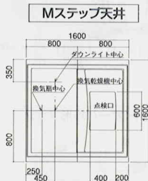
天井伏図
