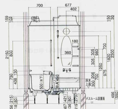
ロセット:オーバル形プラン
