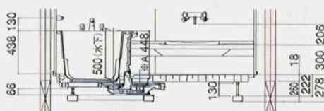
〈階上設置吊り架台仕様〉
