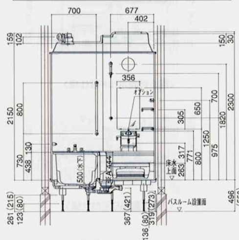
nセット:軟水ピタッチ専用セミロングプラン
