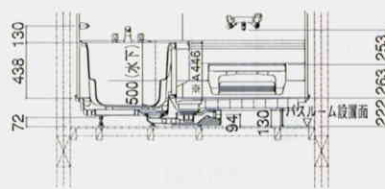
〈階上設置ボルト脚仕様〉
