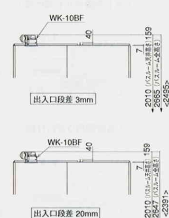
天井断面図
