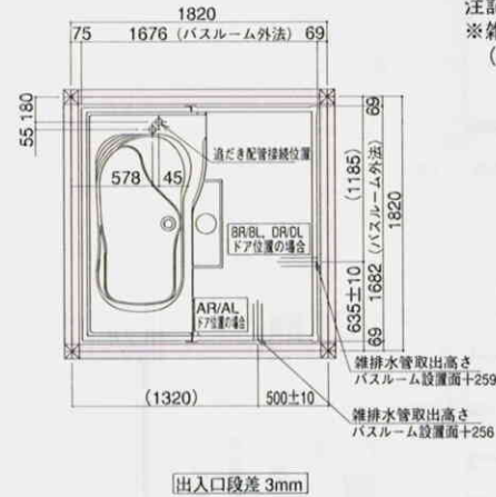
雄排水管取出推奨位置図
