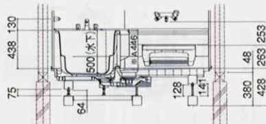
〈1階設置吊り架台仕様〉
