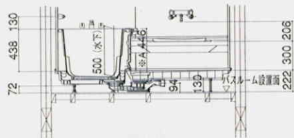
〈階上設置ボルト脚仕様〉
