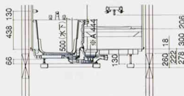
〈階上設置吊り架台仕様〉
