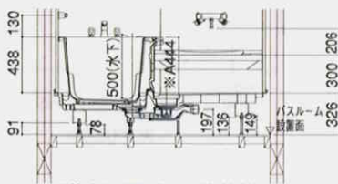
＜階上設置ボルト脚仕様＞
