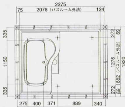
ボルト脚位置図
