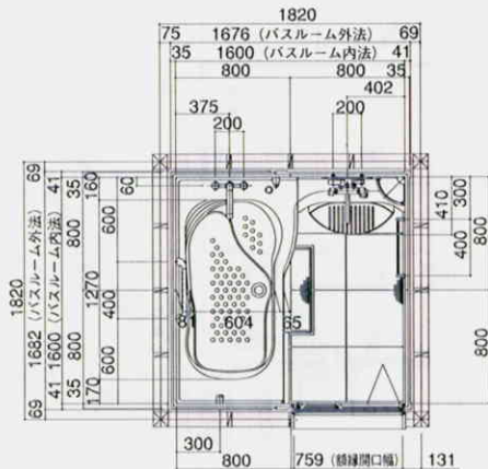
bセット:ロングプラン
