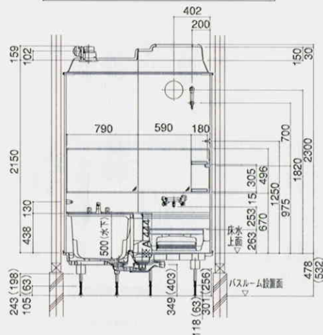
dセット:オーバル形プラン
