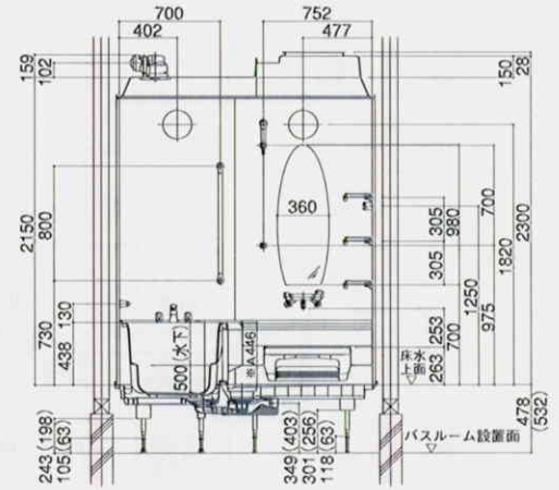
nセット:軟水ピタッチ専用セミロングプラン
