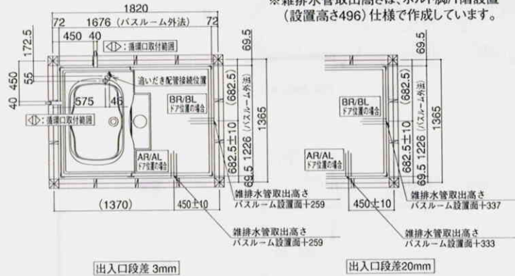
雄排水管取出推奨位置図 循環口取付範囲図
