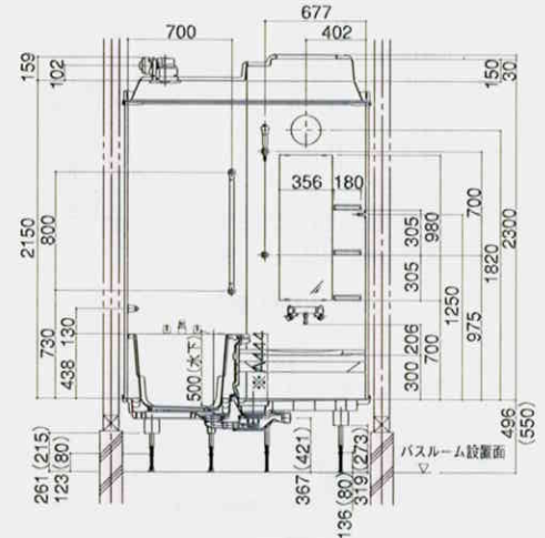
Cセット:横長プラン
