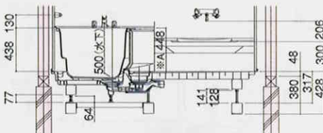
＜1階設置吊り架台仕様＞
