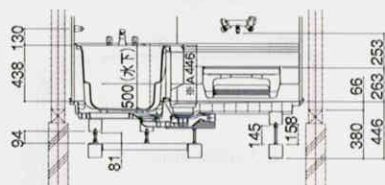
〈1階設置吊り架台仕様〉
