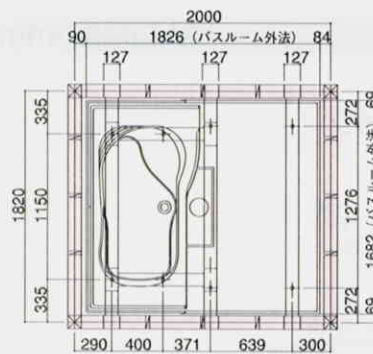
吊り架台位置図
