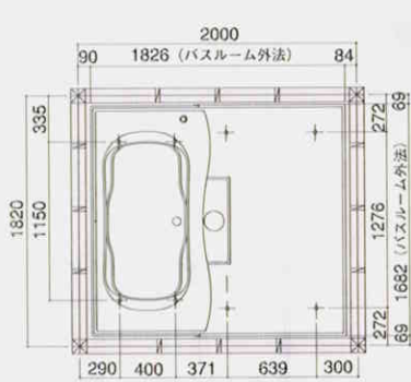
ボルト脚位置図
