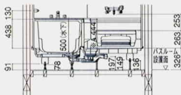
&lt;階上設置ボルト脚仕様&gt;
