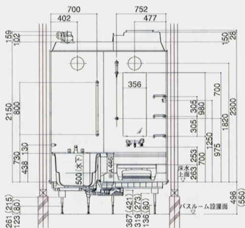
〈1階設置ボルト脚仕様〉
