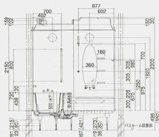
Dセット:オーバル形プラン
