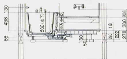
〈階上設置吊り架台仕様〉
