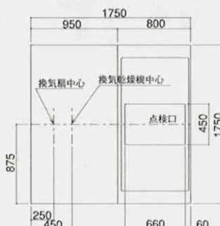
天井伏図
