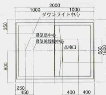
天井伏図
