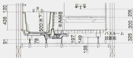
〈階上設置ボルト脚仕様〉
