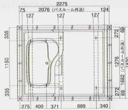
吊り架台位置図
