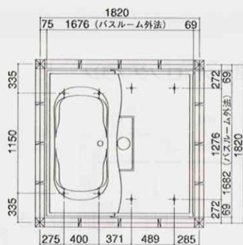
ボルト脚位置図
