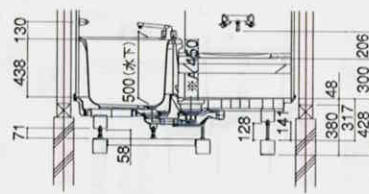
〈1階設置吊り架台仕様〉
