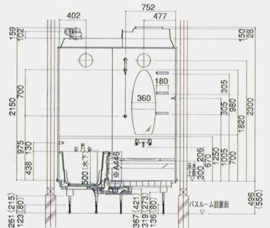
Dセット:オーバル形プラン
