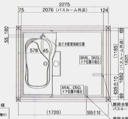
吊り架台位置図
