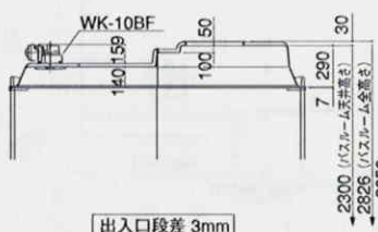
天井断面図
