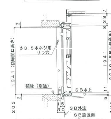
框戸詳細図
