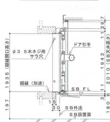
折戸詳細図
