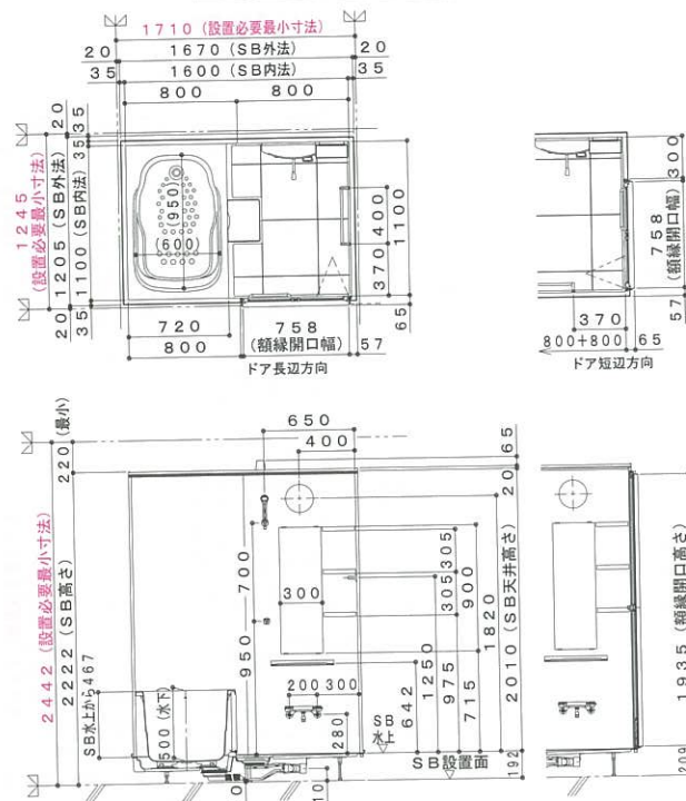
外形寸法図
