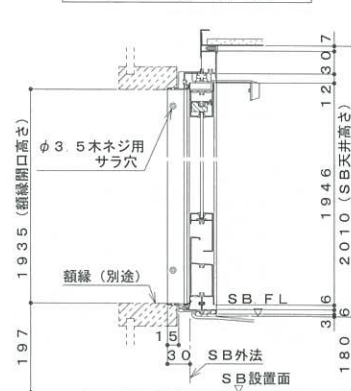
框戸詳細図
