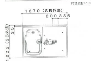
給湯湯ジョイント位置図
