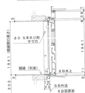
框戸詳細図
