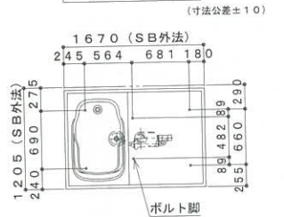
脚位置図
