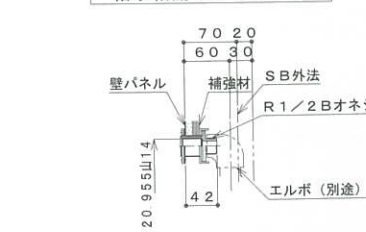
雑排水トラップ部
