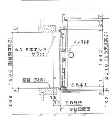
折戸詳細図
