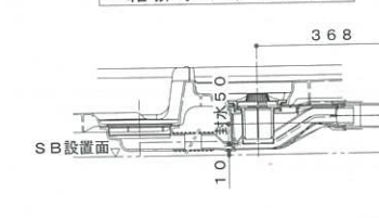
雑排水トラップ部
