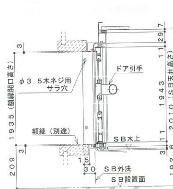
折戸詳細図
