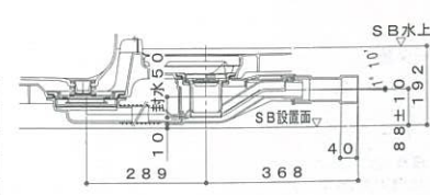
雑排水トラップ部
