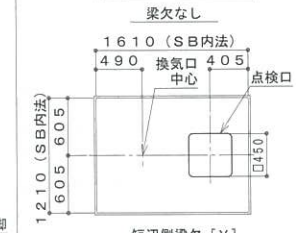
天井伏図
