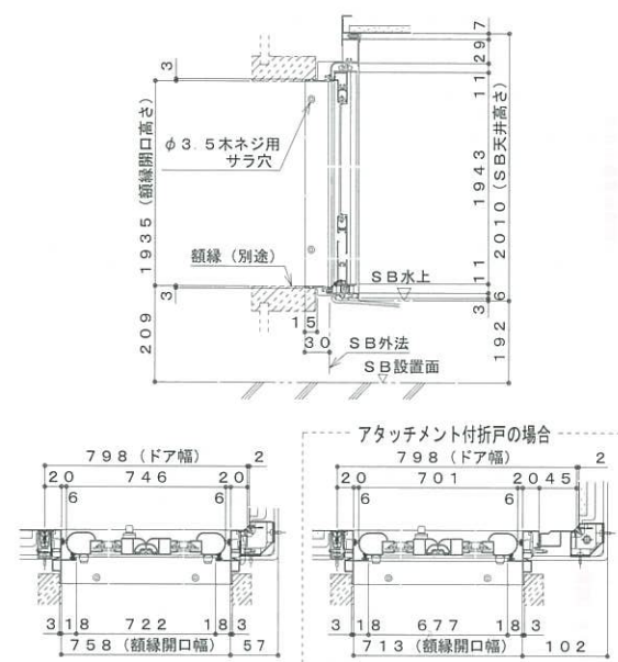
框戸詳細図
