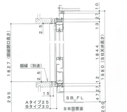
框戸詳細図
