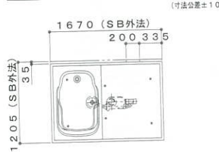
給水湯ジョイント位置図
