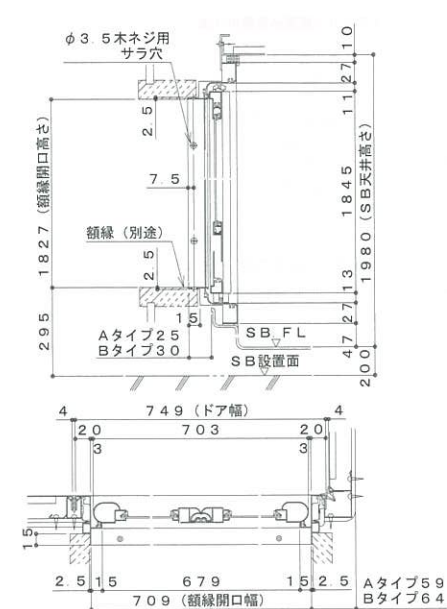
折戸詳細図
