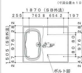
脚位置図
