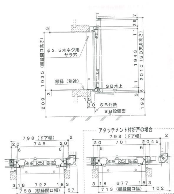
框戸詳細図
