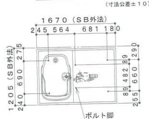
脚位置図
