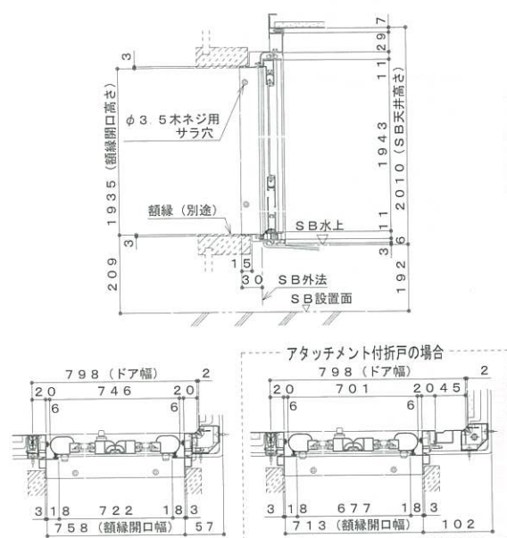
框戸詳細図
