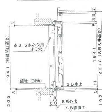
框戸詳細図
