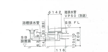
雑排水トラップ部
