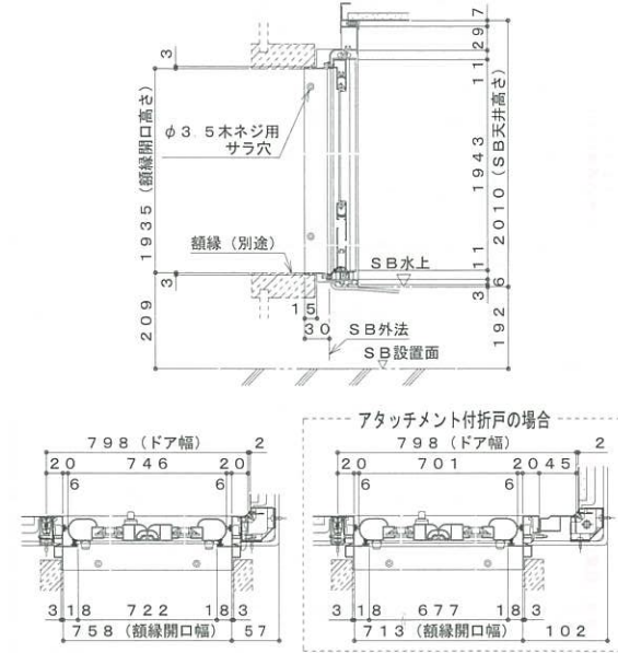
框戸詳細図
