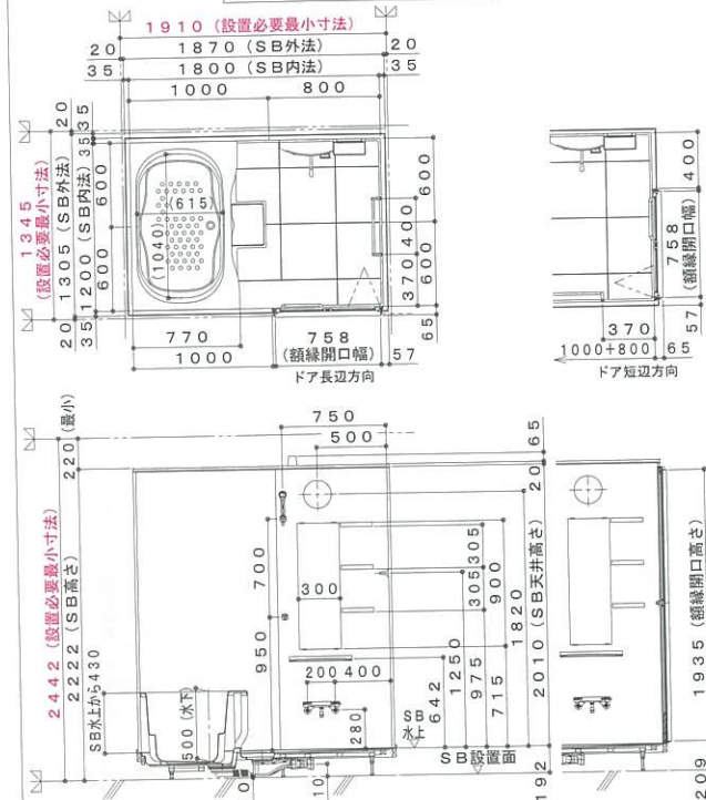
外形寸法図
