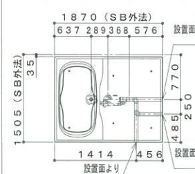
雑排水取り出し推奨位置図
