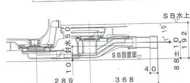
雑排水トラップ部
