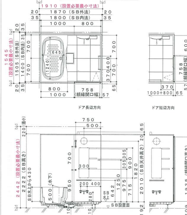
外形寸法図
