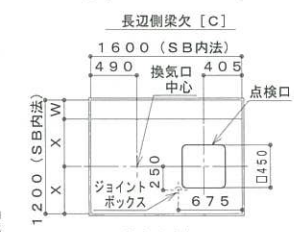
雑排水取り出し推奨位置図
