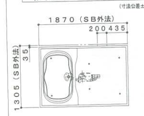
給水湯ジョイント位置図
