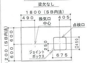
天井伏図
