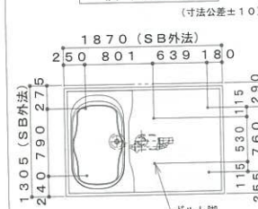
脚位置図
