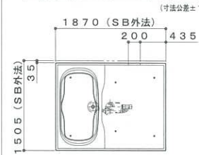
給水湯ジョイント位置図
