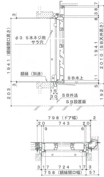
框戸詳細図
