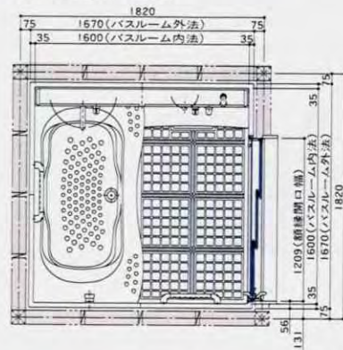
1616(1坪)サイズ・Hカウンター 1階用 〈マベラス・3枚引戸仕様〉
