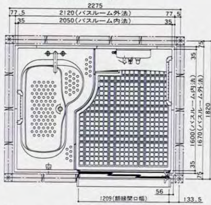
1621(1.25坪)サイズ・Mカウンター 1階用 〈スプレーナ・3枚引戸仕様〉
