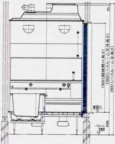
1616(1坪)サイズ・Lカウンター 1階用 〈ジュエロン・框戸仕様〉
