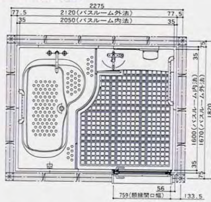
1621(1.25坪)サイズ・Lカウンター 1階用 〈ジュエロン・框戸仕様〉
