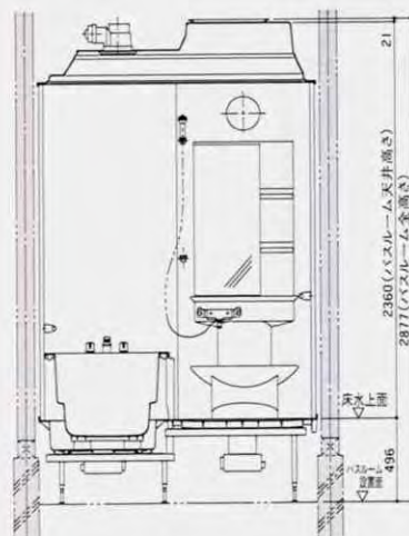
1621(1.25坪)サイズ・収納パネル 1階用 <塩ビ鋼板・折戸仕様>
