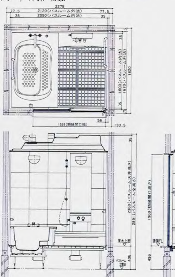
1621(1.25坪)サイズ・Mカウンター／ワイド浴槽 1階用 〈スプレーナ・片引戸仕様〉
