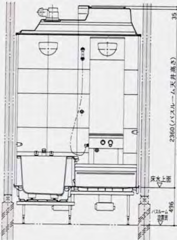
1616(1坪)サイズ・収納パネル 1階用 〈塩ビ鋼板・折戸仕様〉
