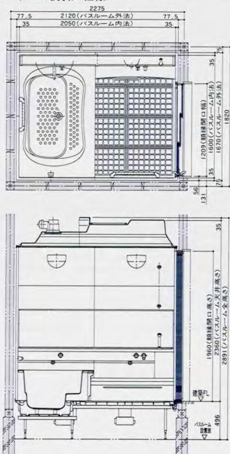
1621(1.25坪)サイズ・Hカウンター／ワイド浴槽 1階用 〈マベラス・3枚引戸仕様〉
