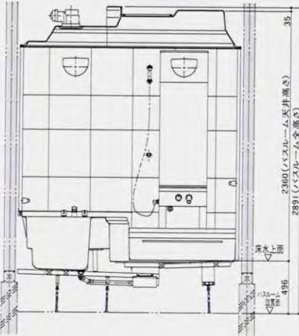
1616(1坪)サイズ・Lカウンター 1階用 〈ジュエロン・框戸仕様〉
