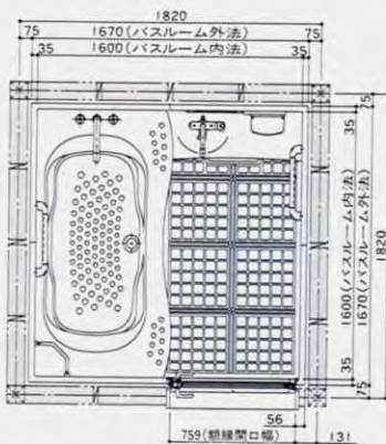
1616(1坪)サイズ・Lカウンター 1階用 〈ジュエロン・框戸仕様〉
