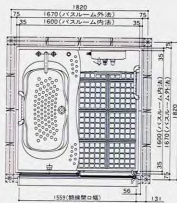
1616(1坪)サイズ・Mカウンター 1階用 〈スプレーナ・片引戸仕様〉
