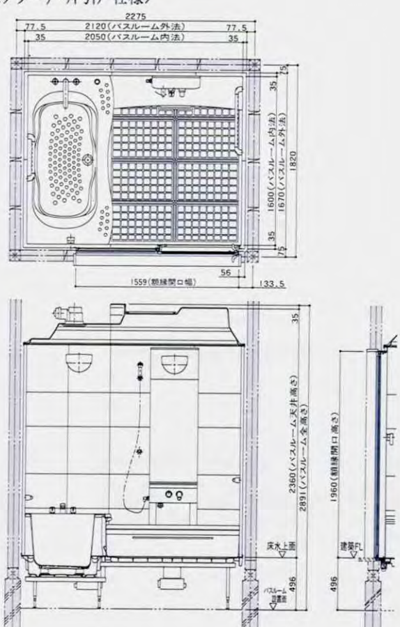
1621(1.25坪)サイズ・Mカウンター 1階用 〈スプレーナ・片引戸仕様〉
