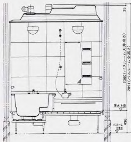
1621(1.25坪)サイズ・Lカウンター 1階用 <ジュエロン・框戸仕様>
