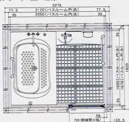
1621(1.25坪)サイズ・Lカウンター／ワイド浴槽 1階用 <スプレーナ・框戸仕様>
