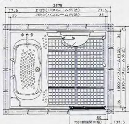
1621(1.25坪)サイズ・収納パネル 1階用 <塩ビ鋼板・折戸仕様>
