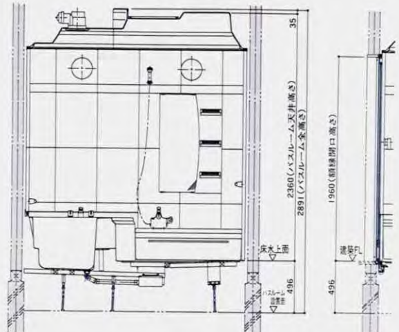
1616(1坪)サイズ・収納パネル 1階用 〈塩ビ鋼板・折戸仕様〉
