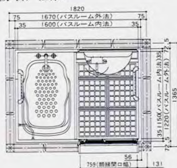
1216(0.75坪)サイズ・収納パネル 1階用 <塩ビ鋼板・折戸仕様>
