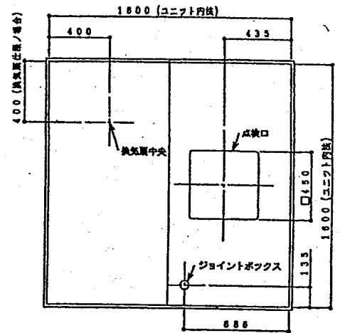
天井伏図
