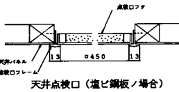
天井点検口 (蓋ノ鋼板ノ場合)
