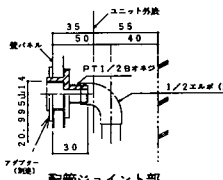
壁パネル縦断面
