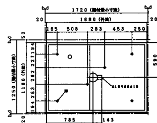
雜排水、床下腳位置圖
