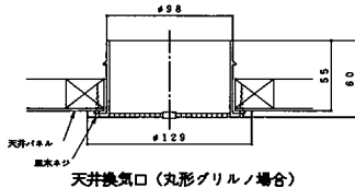
天井換気口 (丸形グリルノ場合)
