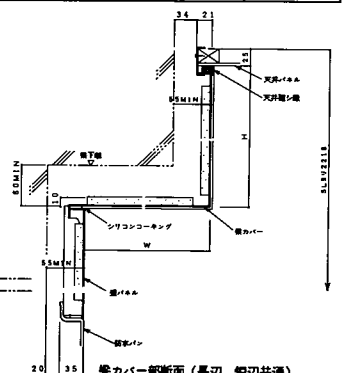
梁カバー部断面(長辺、短辺共通)
