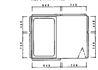
パネル割図
