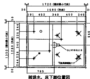
雑排水、床下脚位置図
