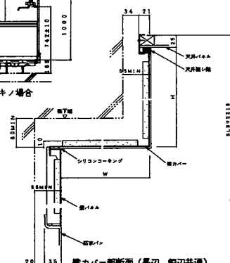
梁カバー部断面 (長辺、短辺共通)
