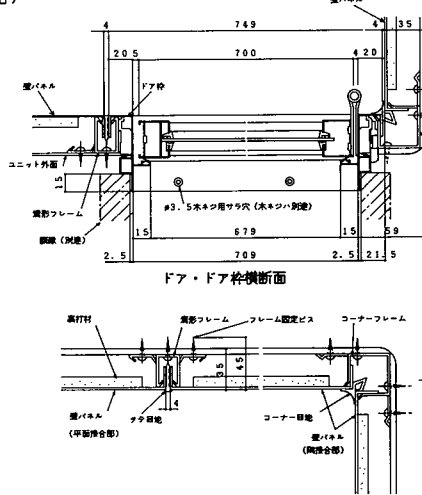
壁パネル横断面
