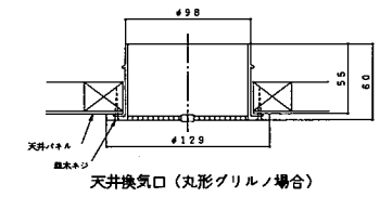
天井換気口 (丸形グリルノ場合)
