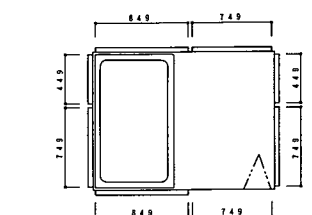
パネル割図
