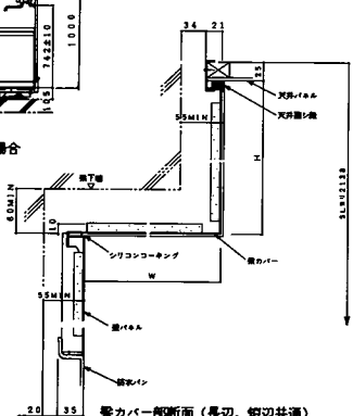
梁欠キ部断面 (長辺、短辺共通)
