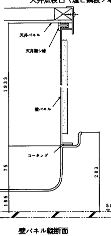
壁パネル縦断面
