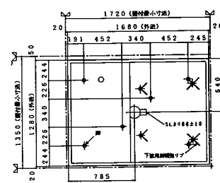
雑排水、床下脚位置図
