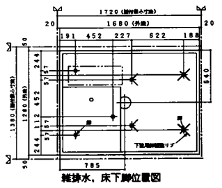
雑排水、床下脚位置図
