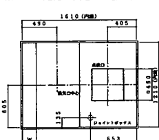
短辺梁切欠キ天井換気口
