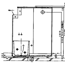
短辺梁欠キノ場合
