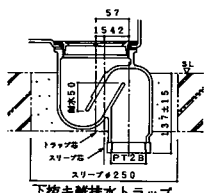
下排水雑排水トラップ
