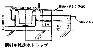
横引き雑排水トラップ
