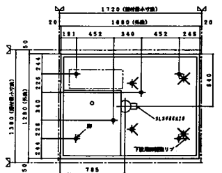
縦排水、床下脚位置図
