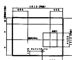
長辺梁切欠キ天井伏図
