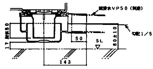
横引キ排水トラップ
