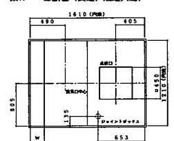
短辺梁欠き天井伏図
