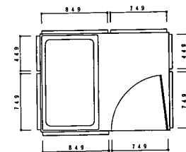
パネル割図
