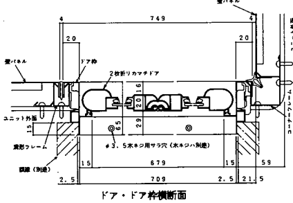
ドア・ドア枠横断面
