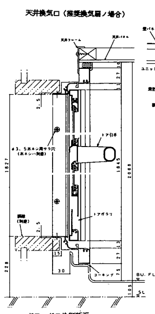
ドア・ドア枠縦断面
