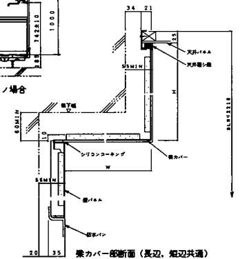
梁欠き部断面 (長辺、短辺共通)
