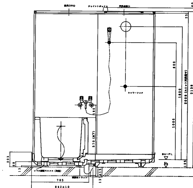
断面A-A
