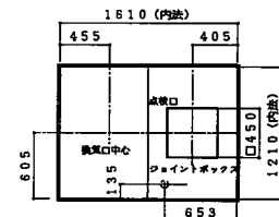
天井伏図
