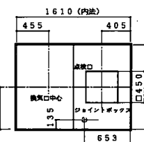
天井換気口
