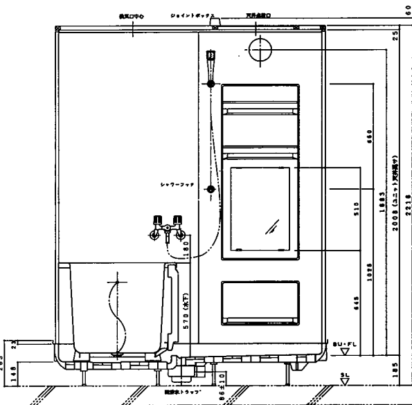
ドア長辺方向
