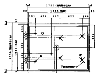
雑排水、床下脚位置図
