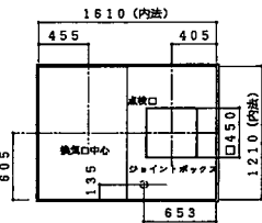
天井伏図
