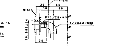
配管ジョイント部
