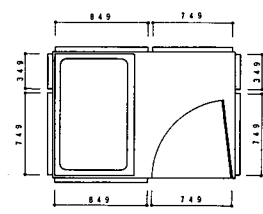
パネル割区
