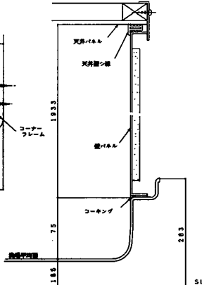
壁パネル断面
