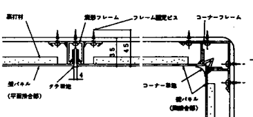
壁パネル断面
