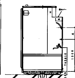
長辺梁欠キノ場合
