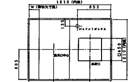
短辺梁欠き天井伏図
