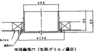
断面 A-A
