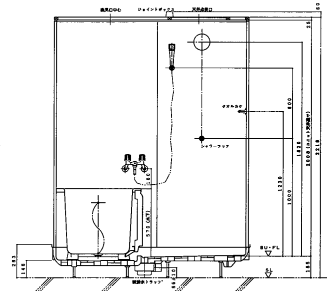
断面 A-A
