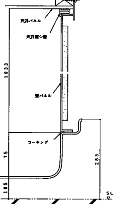
壁パネル縦断面
