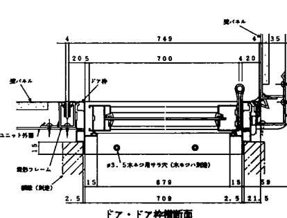
ドア・ドア枠断面
