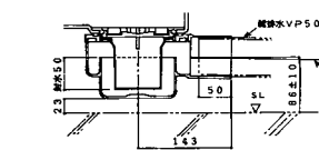
横引キ排水トラップ
