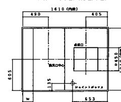
短辺梁切欠キ天井伏図
