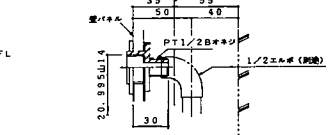
配管ジョイント部
