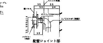
配管ジョイント部
