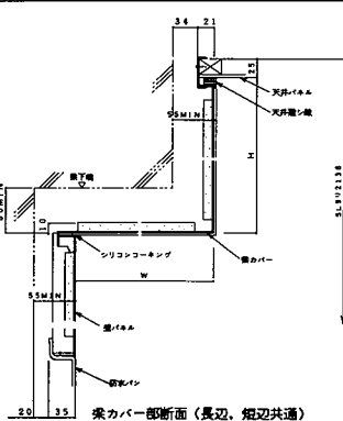
梁切欠き部断面 (長辺、短辺共通)
