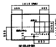
天井伏図
