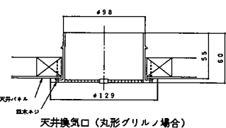
天井換気口(丸形グリルノ場合)
