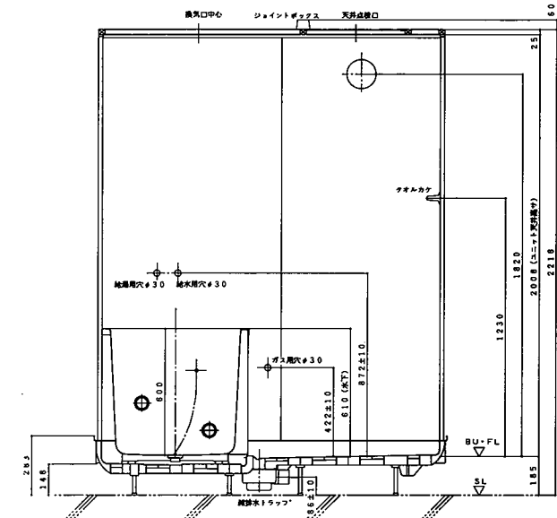
断面 A-A
