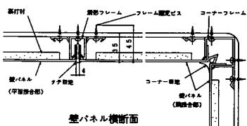
壁パネル横断面
