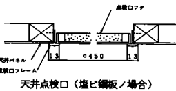
天井点検口 (塩ビ板ノ場合)
