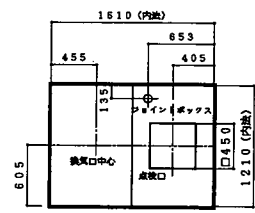
天井伏図
