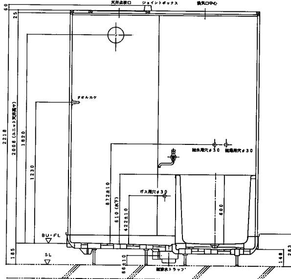
断面A-A
