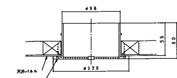
天井換気口（丸形グリルの場合）
