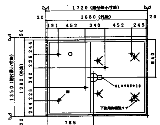
排水水、床下脚位置図
