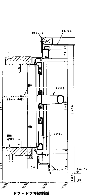
ドア・ドア枠縦断面
