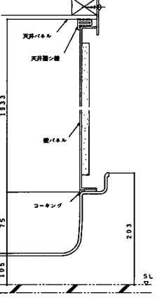
壁パネル縦断面
