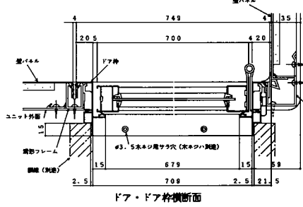
ドア・ドア枠横断面
