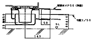
横引き排水水トラップ
