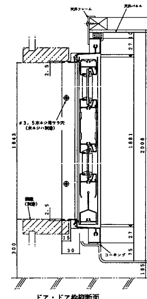
ドア・ドア枠断面
