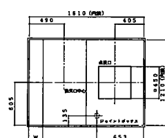
短辺梁切欠キ天井伏図
