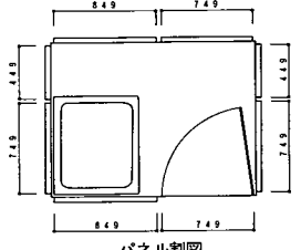
パネル割図
