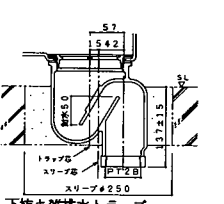
下排水排水トラップ
