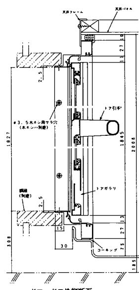
ドア・ドア枠断面
