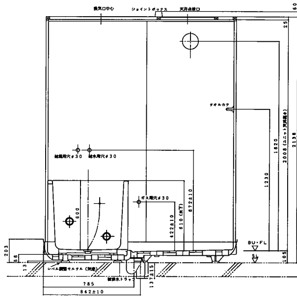
断面 A-A
