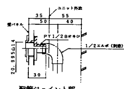
配管ジョイント部
