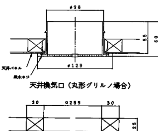
断面A-A
