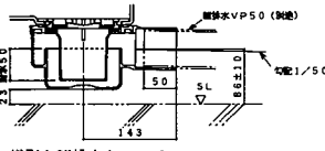
壁パネル縦断面
