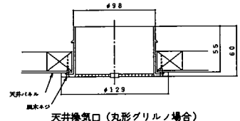
天井換気口 (丸形グリルノ場合)
