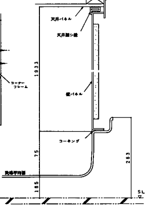
壁パネル縦断面
