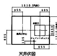
天井伏図
