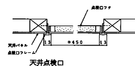
天井点検口
