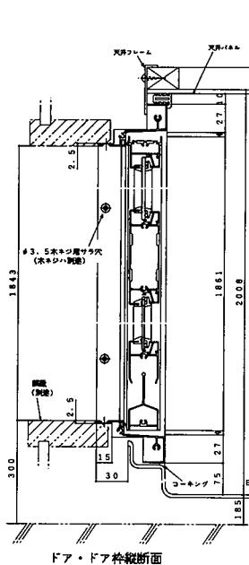
ドア・ドア枠縦断面
