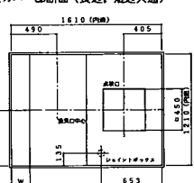
短辺梁欠キ天井伏図
