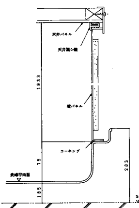
壁パネル縦断面
