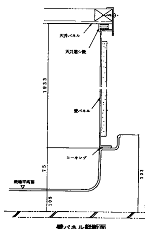
壁パネル縦断面
