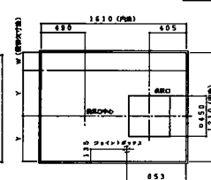
長辺梁欠き天井伏図
