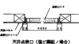
天井点検口 (塩ビ鋼板ノ場合)
