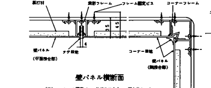
壁パネル横断面
