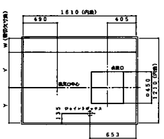
長辺梁切欠キ天井伏図
