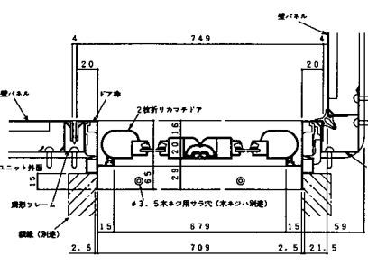
ドア・ドア枠横断面
