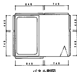
パネル割図
