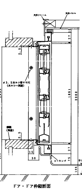
ドア・ドア枠縦断面
