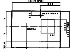
長辺梁欠き天井伏図
