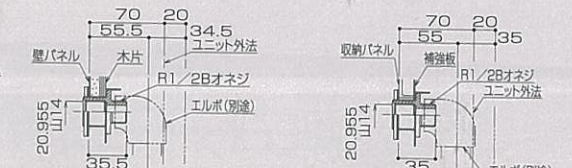
壁パネル取付洗場・浴槽水栓部 給水・給湯ジョイント
