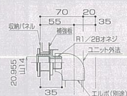
収納パネル取付洗場水栓部 給水・給湯ジョイント
