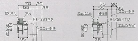
壁パネル取付洗場・浴槽水栓部 給水・給湯ジョイント
