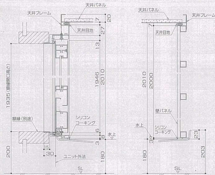
ドア・ドア枠縦断面<框戸>
