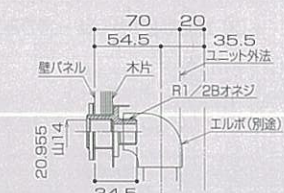
壁パネル取付洗場・浴槽水栓部 給水・給湯ジョイント
