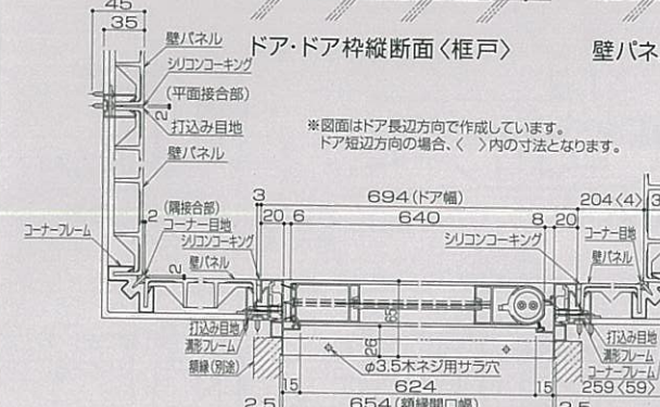
壁パネル、ドア・ドア枠横断面<框戸>
