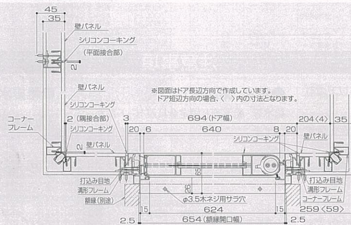
壁パネル、ドア・ドア枠横断面<框戸>
