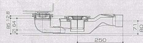
雑排水トラップ
