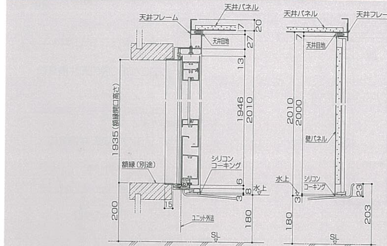
ドア・ドア枠縦断面<框戸>
