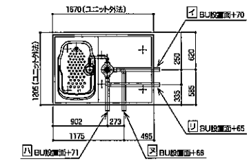
1116雑排水位置図
