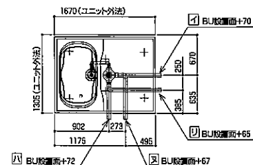
1216雑排水位置図
