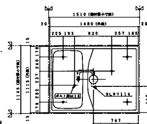
雑排水・床下脚位置図
