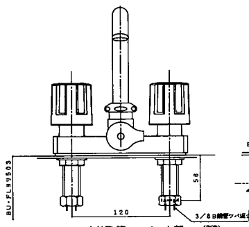
シャワーバス水栓配管ジョイント部 (別図)
