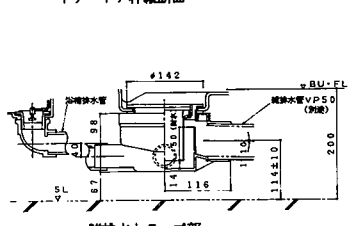
雑排水トラップ部
