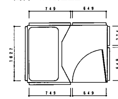
パネリ割図
