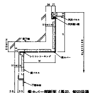
柔カバ一部断面（長辺、短辺共通）
