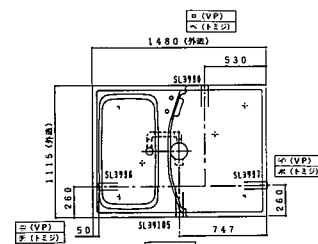
配管図
