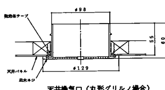
天井換気口（丸形グリルノ場合）
