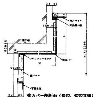
梁カバー部断面 (長辺、短辺共通)
