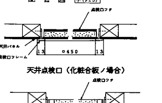
天井換気口 (化粧板/場合)
