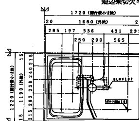
雑排水、床下脚位置図
