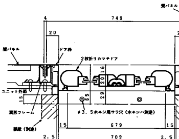
ドア・ドア枠断面 (折り戸)
