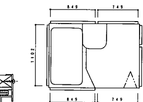
パネル割図
