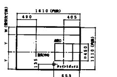
長辺梁切欠き天井伏図
