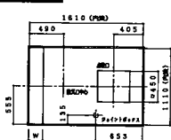
短辺梁切欠き天井伏図
