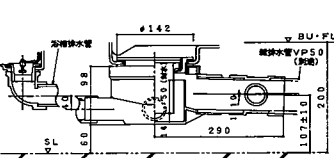
雑排水トラップ部 (1/4)
