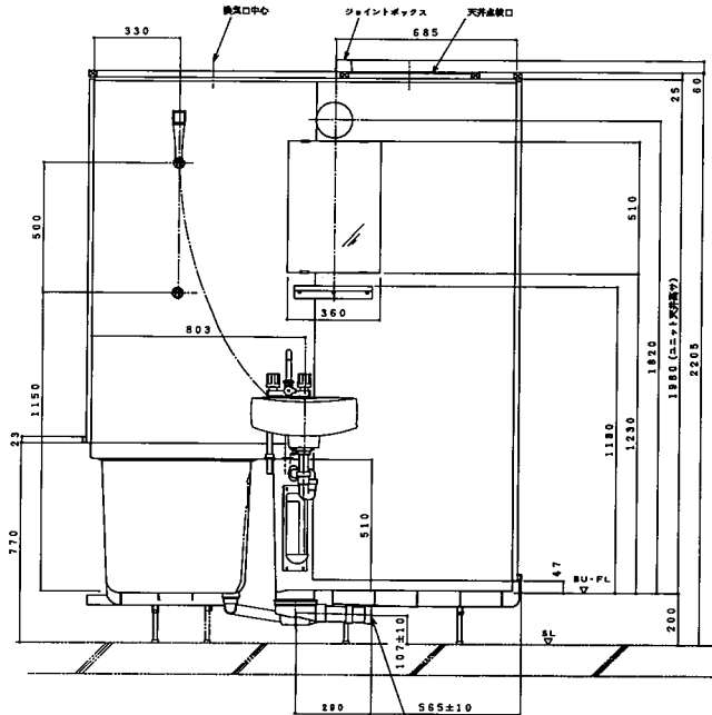
断面 A-A
