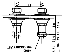
給水、給湯管ジョイント部
