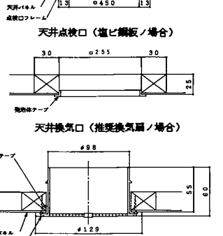
天井換気口 (丸形グリル/場合)
