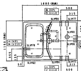
配管図
