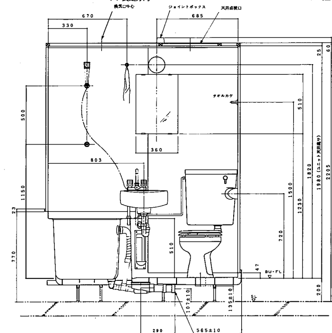
断面 A-A
