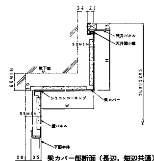
梁カバー部断面 (長辺, 短辺共通)
