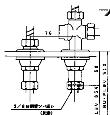
壁パネル縦断面
