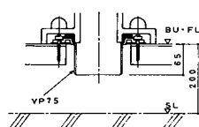
壁パネル縦断面
