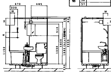
梁切欠きタイプ寸法表
