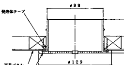
天井換気口 (丸形グリルノ場合)
