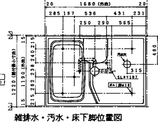
雑排水・汚水・床下脚位置図
