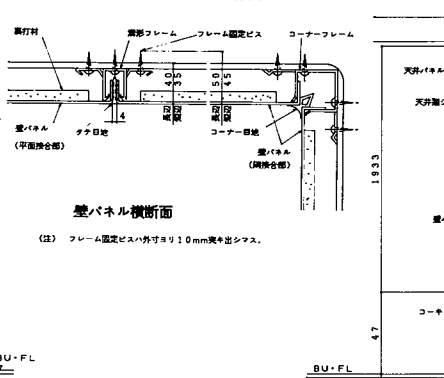
壁パネル横断面
