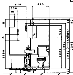
梁切欠きタイプ寸法表
