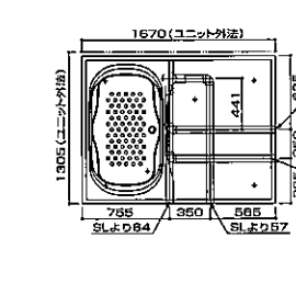
1117床下脚位置図
