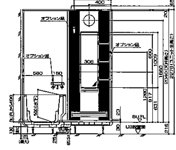
1117収納パネルタイプ
