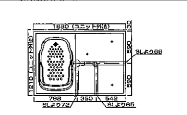
1116雑排水位置図
