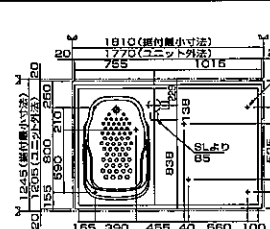
1117床下脚位置図
