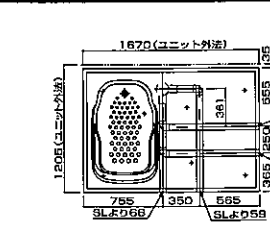
1116雑排水位置図
