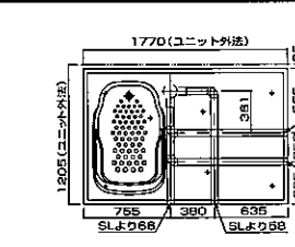
1117雑排水位置図
