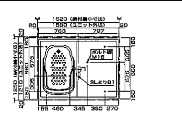
1115床下脚位置図
