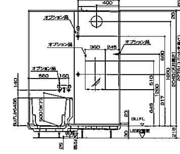
1117全面壁タイプ
