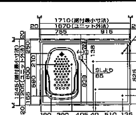
1116床下脚位置図
