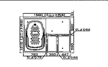
1115雑排水位置図
