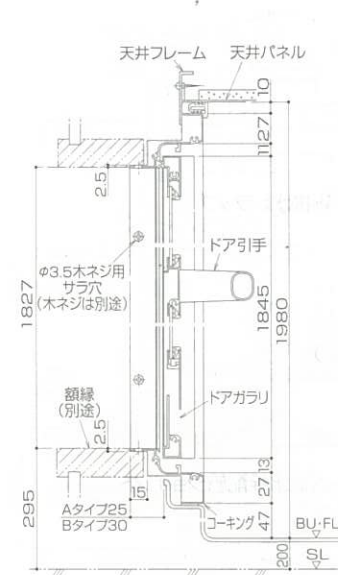
ドア・ドア枠縦断面<折戸>
