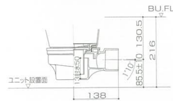
雑排水トラップ
