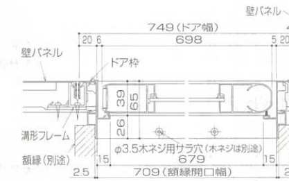
ドア・ドア枠横断面<框戸>
