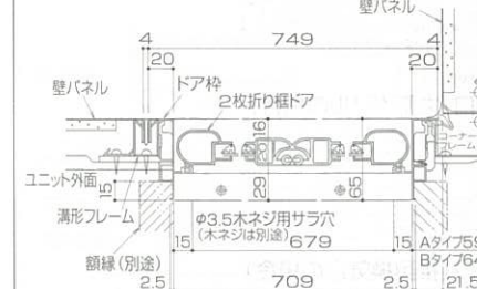
ドア・ドア枠横断面<折戸>
