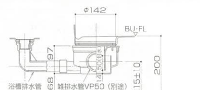
雑排水トラップ
