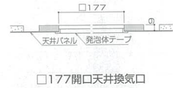
177開口天井換気口
