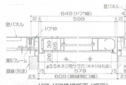
ドア・ドア枠横断面<框戸>
