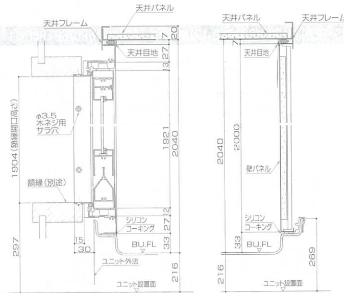
ドア・ドア枠縦断面<框戸>
