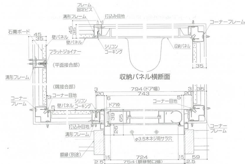
壁パネル・ドア・ドア枠横断面<框戸>
