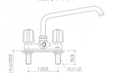
シャワー・バス水栓配管ジョイント
