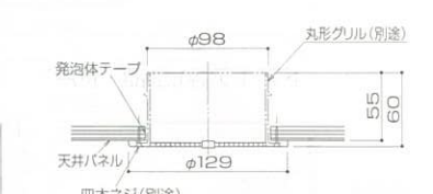
天井換気口 (丸形グリルの場合)
