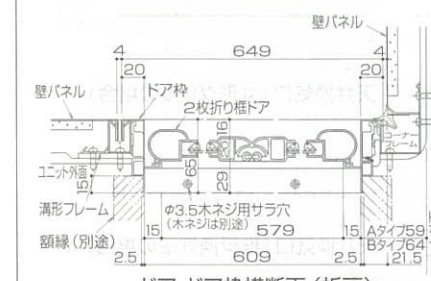
ドア・ドア枠横断面<折戸>
