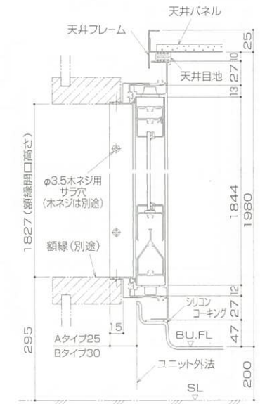
ドア・ドア枠縦断面<框戸>
