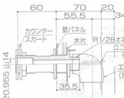
カウンター取付洗場水栓部 給水・給湯ジョイント
