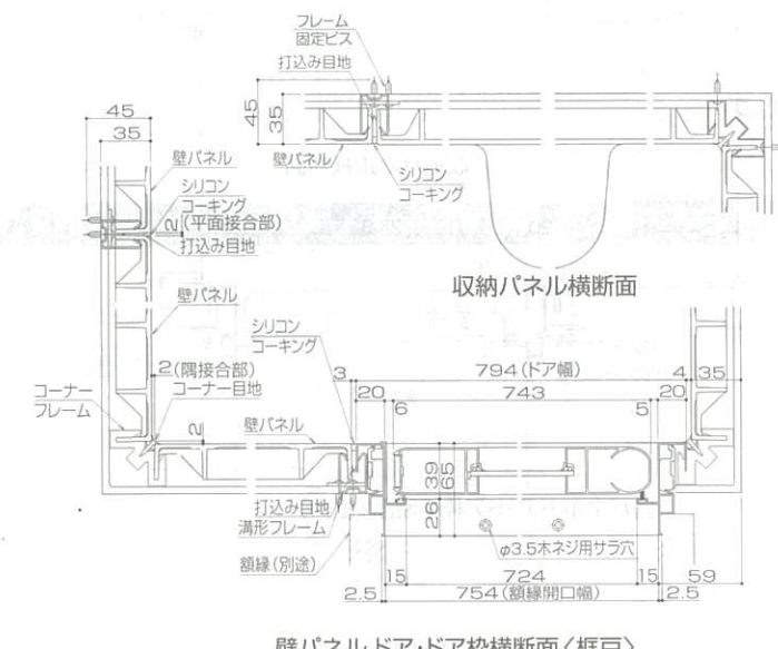
壁パネル、ドア・ドア枠横断面<框戸>
