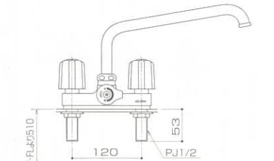
シャワー・バス水栓配管ジョイント
