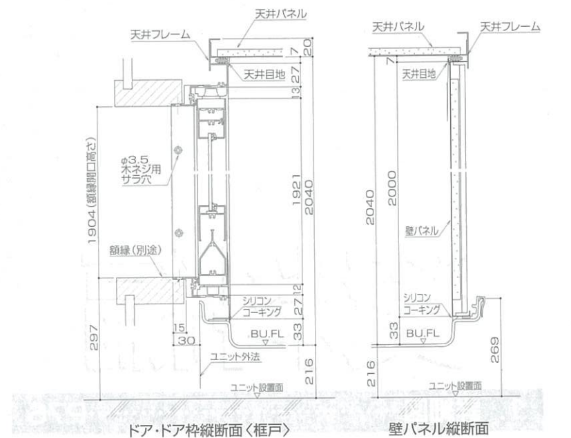
ドア・ドア枠縦断面<框戸>
