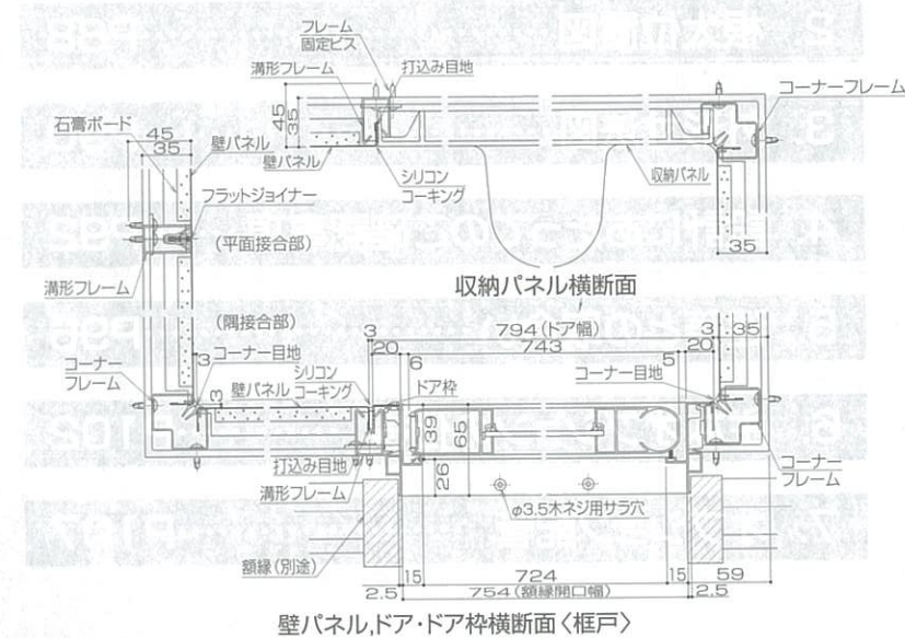
壁パネル、ドア・ドア枠横断面<框戸>
