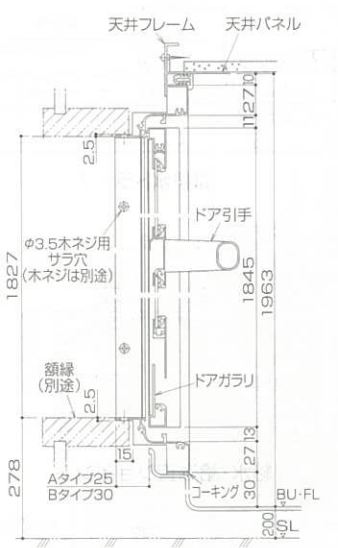
ドア・ドア枠縦断面<折戸>
