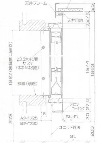
ドア・ドア枠縦断面<框戸>
