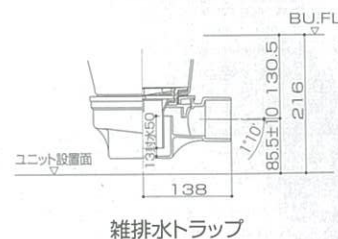
雑排水トラップ
