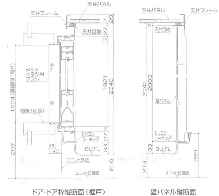
ドア・ドア枠縦断面<框戸>
