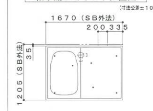
給水湯ジョイント位置図
