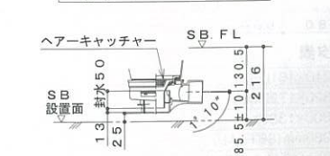
雑排水トラップ部
