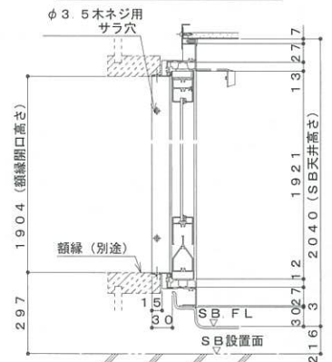
框戸詳細図
