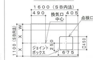
梁欠寸法表
