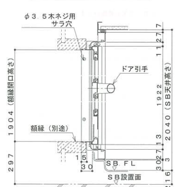
折戸詳細図
