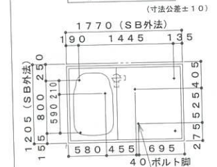
脚位置図
