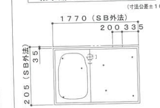
給水湯ジョイント位置図
