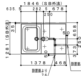
雑排水取り出し推奨位置図
