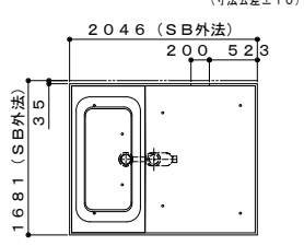
雑排水取り出し推奨位置図
