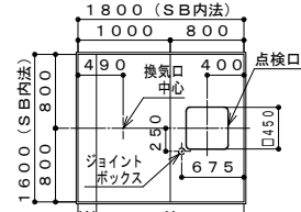
長辺側梁欠[C]
