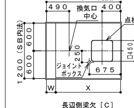
長辺側梁欠[C]
