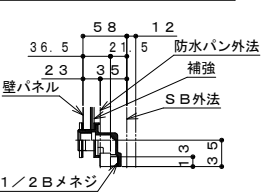
雑排水トラップ部
