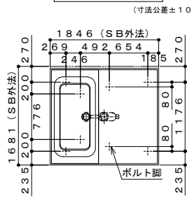
給水湯ジョイント位置図
