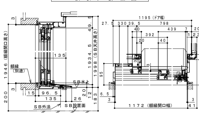
2 枚 引 戸 詳 細 図
