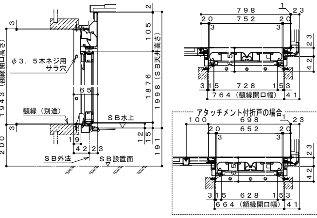
開き戸詳細図
