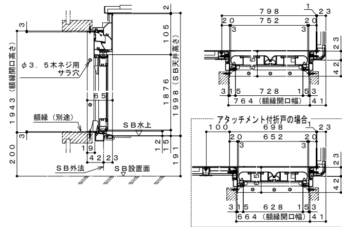
開き戸詳細図
