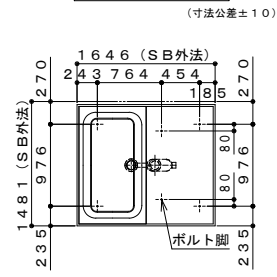
脚位置図
