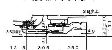
雑排水トラップ部
