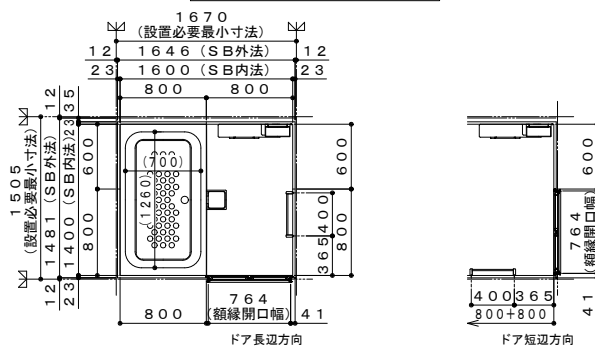
外形寸法図
