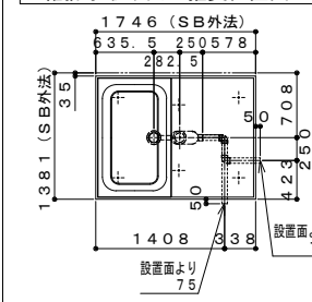
雑排水取り出し推奨位置図
