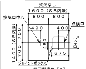
天井伏図
