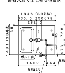
雑排水取り出し推奨位置図
