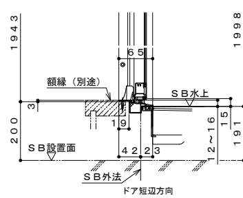
開 き 戸 詳 細 図
