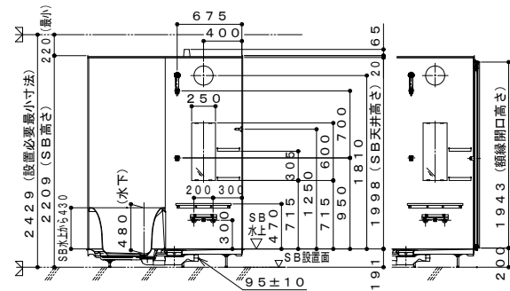
脚位置図
