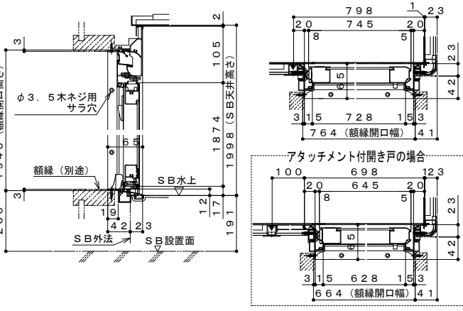
2枚引戸詳細図
