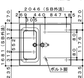
給水湯ジョイント位置図
