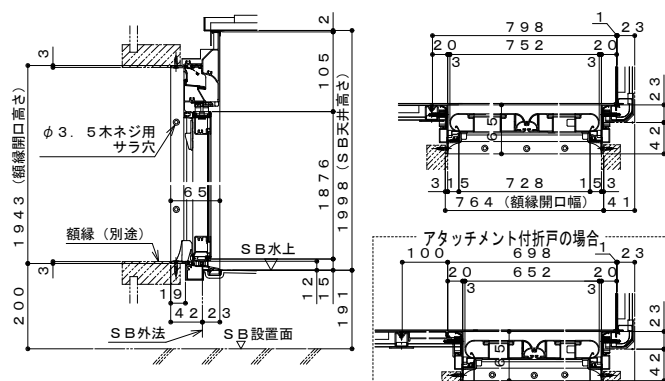
折戸詳細図
