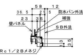
雑排水トラップ部
