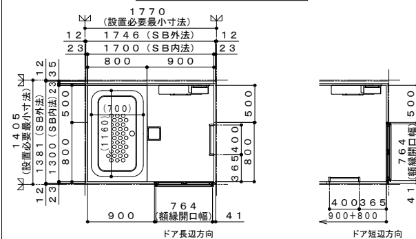
外形寸法図
