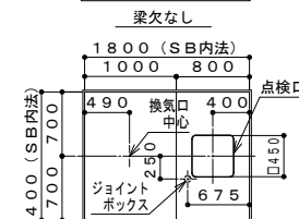
短辺側梁欠[Y]
