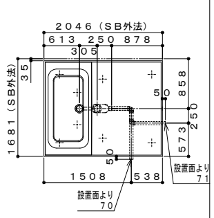
雑排水取り出し推奨位置図
