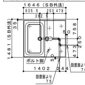
雑排水取り出し推奨位置図
