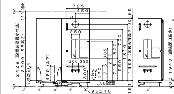
脚位置図
