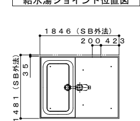
給水湯ジョイント位置図
