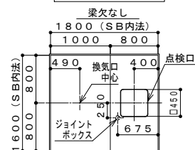
短辺側梁欠[Y]
