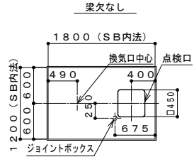
短辺側梁欠[Y]
