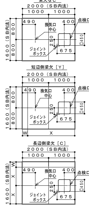
天井伏図
