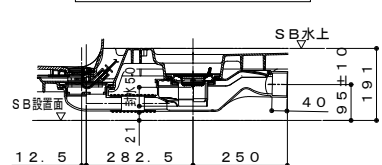
雑排水トラップ部
