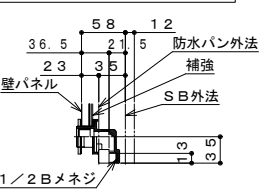
雑排水トラップ部
