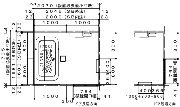
外形寸法図
