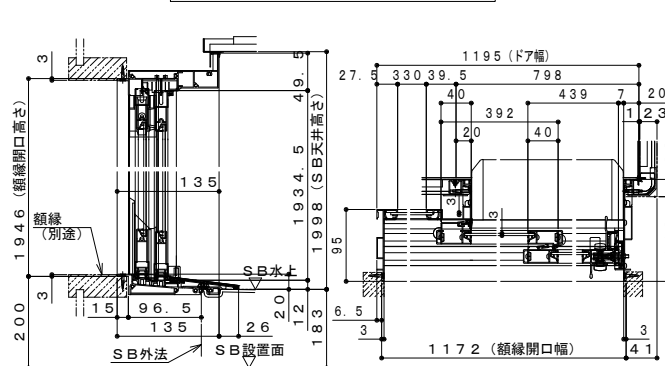
2枚引戸詳細図
