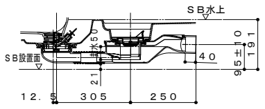
雑排水トラップ部
