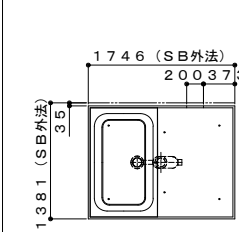
給水湯ジョイント位置図
