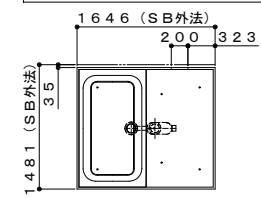
給水湯ジョイント位置図
