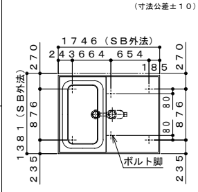
給水湯ジョイント位置図
