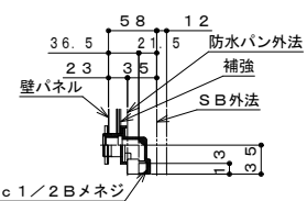
雑排水トラップ部
