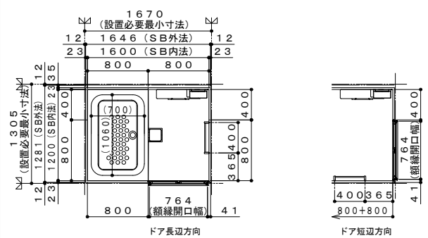
外形寸法図
