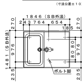
給水湯ジョイント位置図
