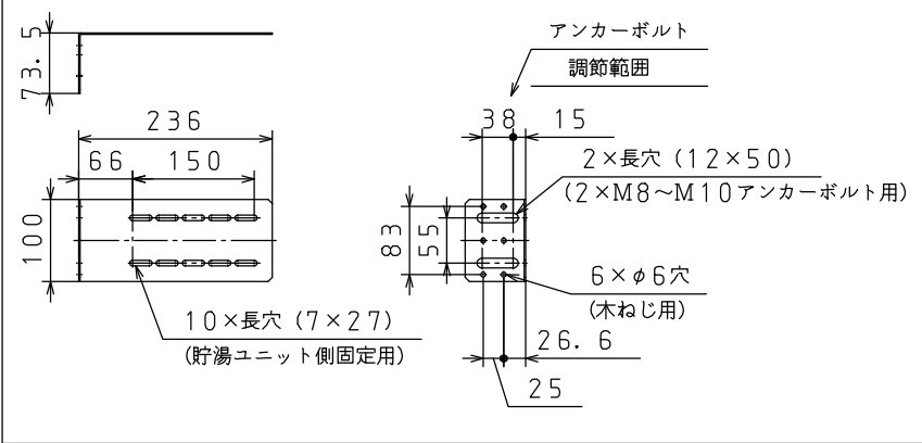
壁固定金具 外形寸法図 (本体に1個付属)
