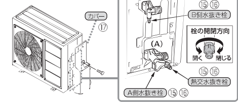
■ヒートポンプユニット
