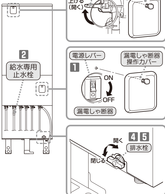
■ 貯湯ユニット (図は370Lタイプ)
