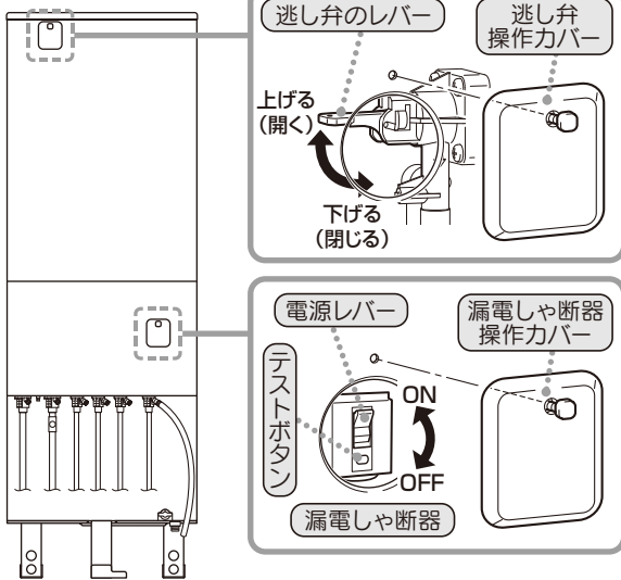
■ 貯湯ユニット (図は370Lタイプ)
