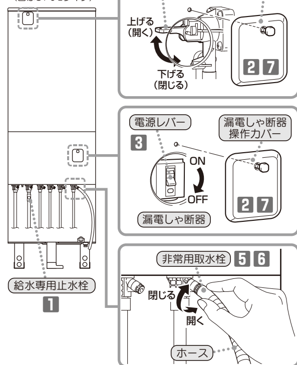
■貯湯ユニット (図は370Lタイプ)
