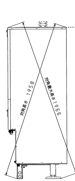
右側面
