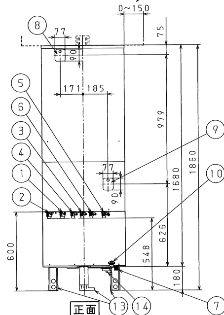
正面
