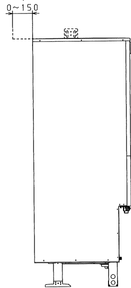
左側面
