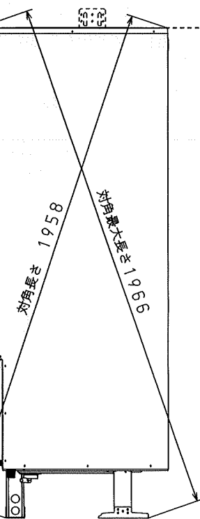
右側面
