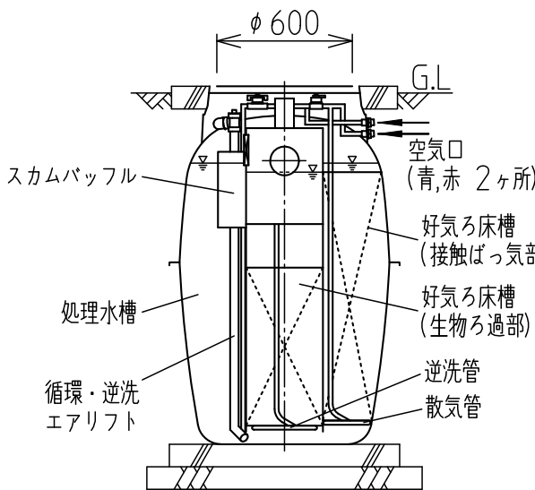
B-B'断面図
