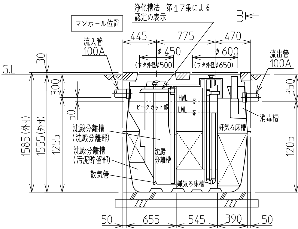
A-A'断面図
