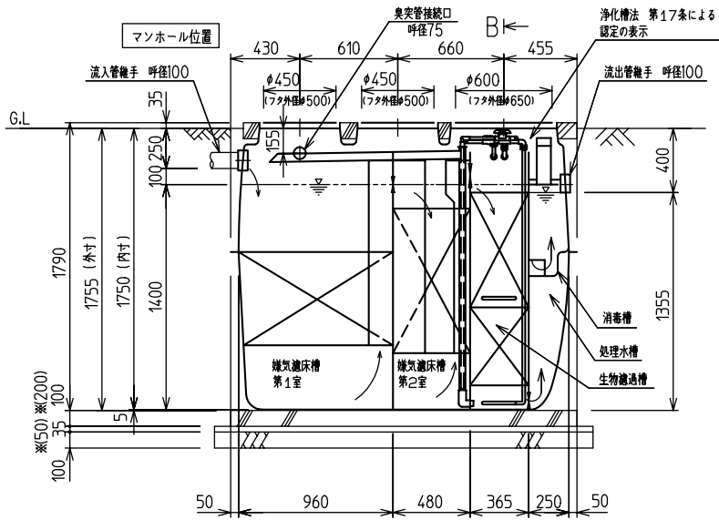
A-A'断面図
