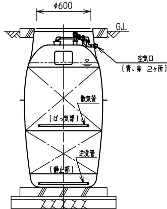
B-B'断面図
