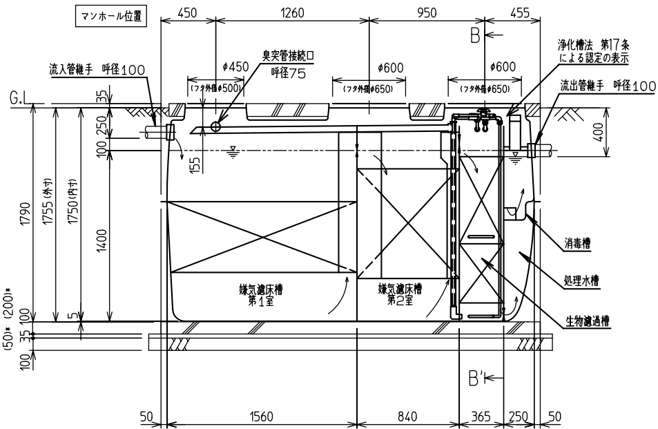
A-A'断面図
