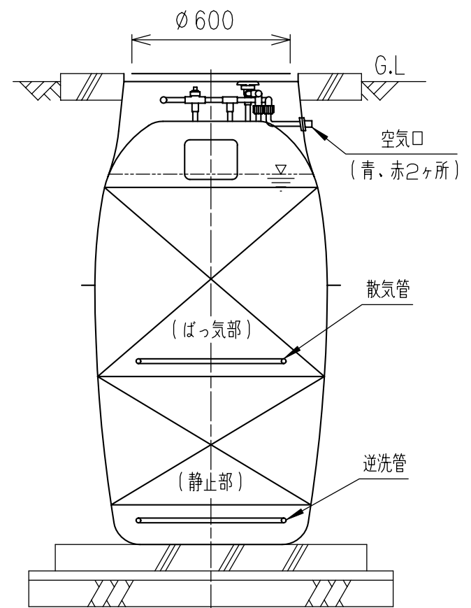
B-B'断面図
