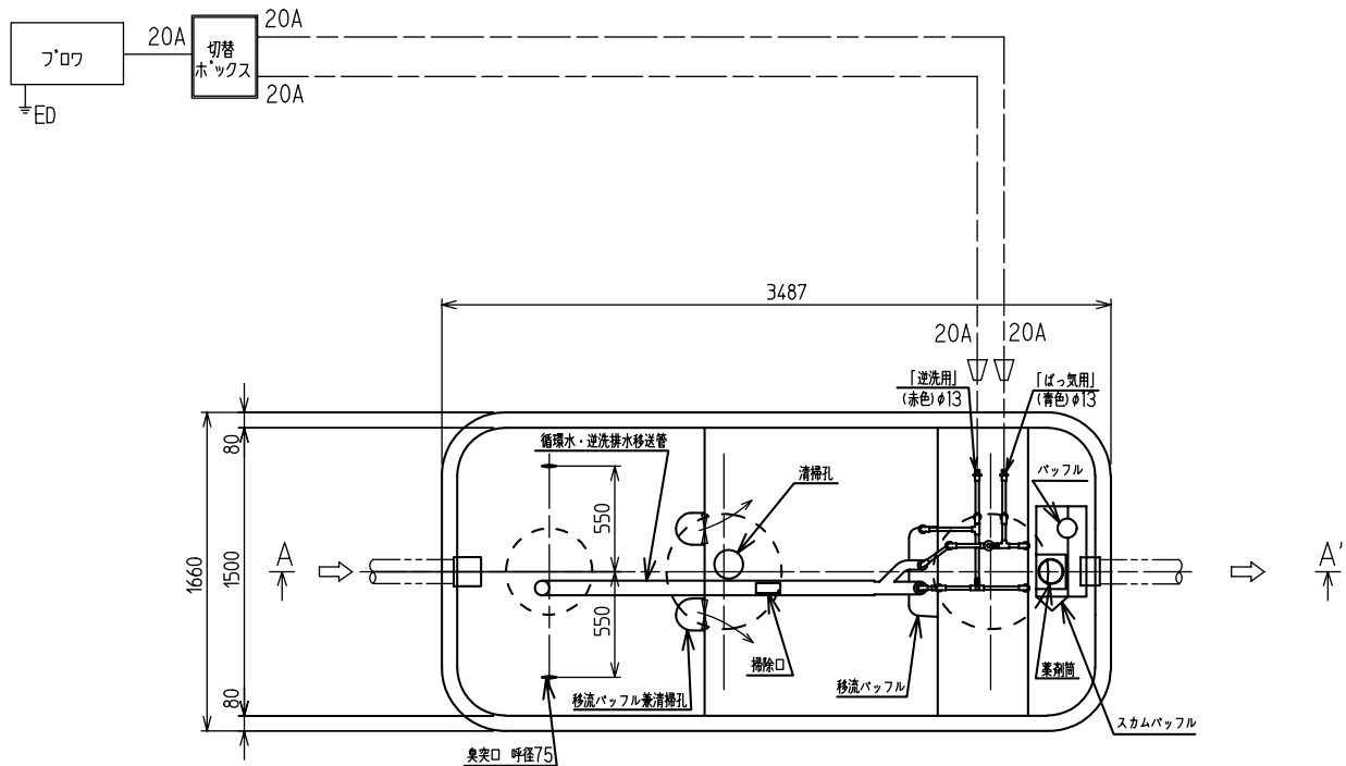
平面図
