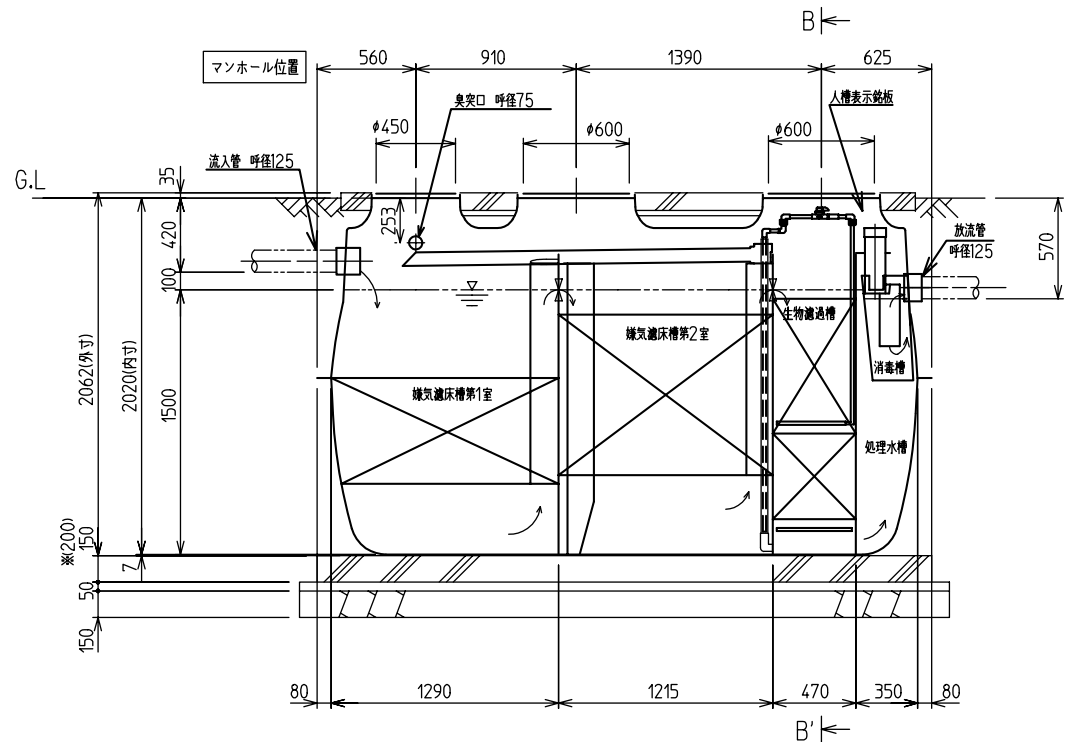
A-A'断面図
