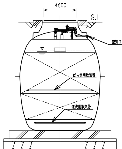
B-B'断面図
