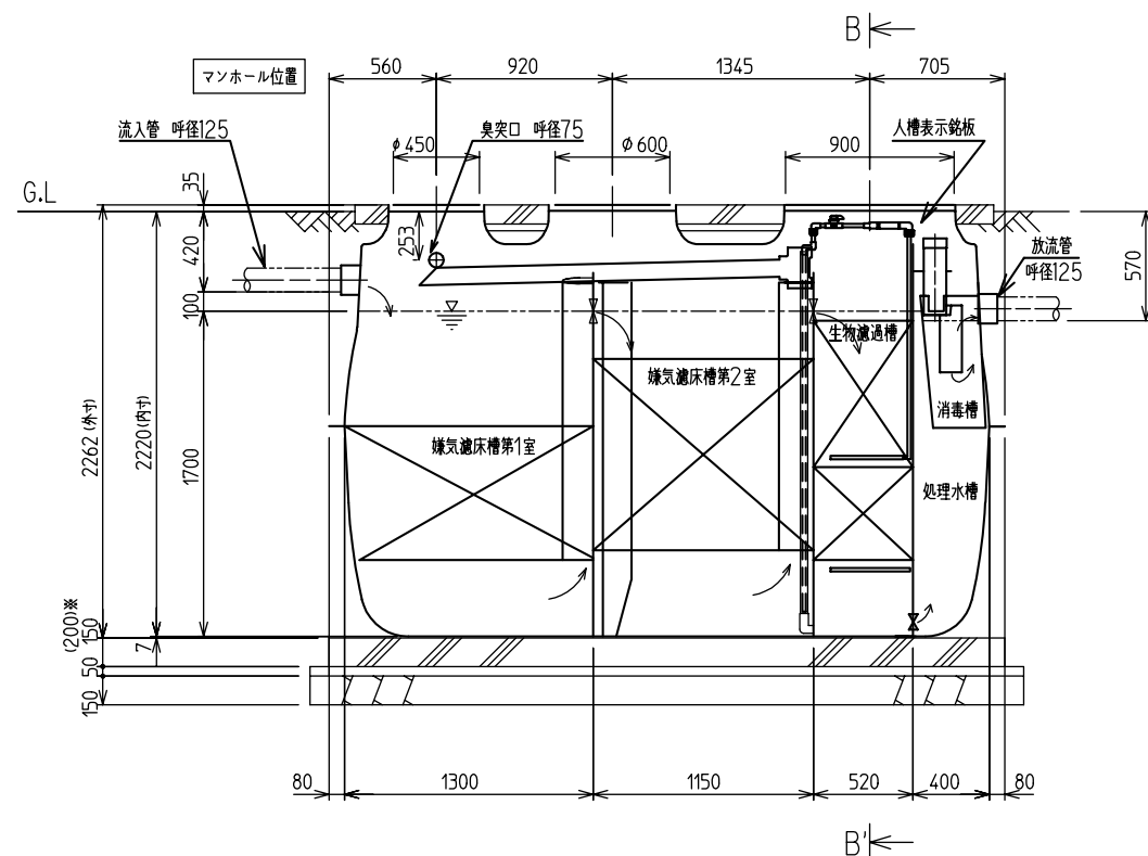
A-A'断面图
