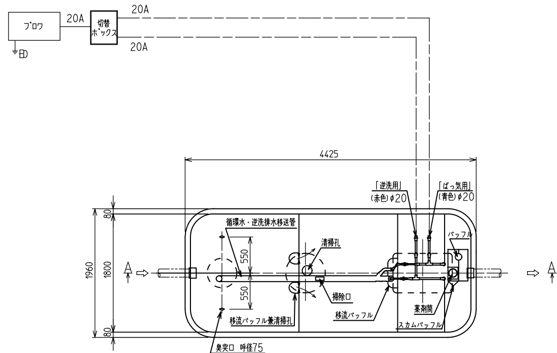
平面图
