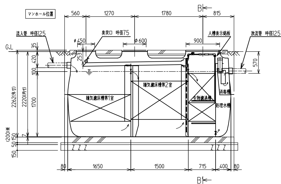
A-A'断面图
