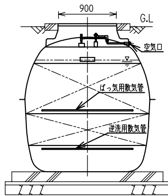
B-B'断面図
