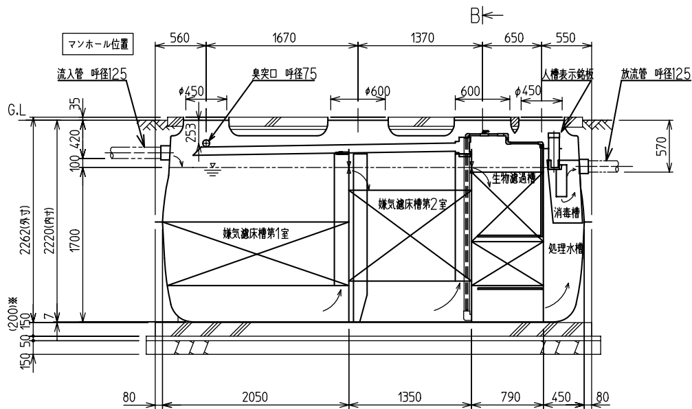
A-A'断面図
