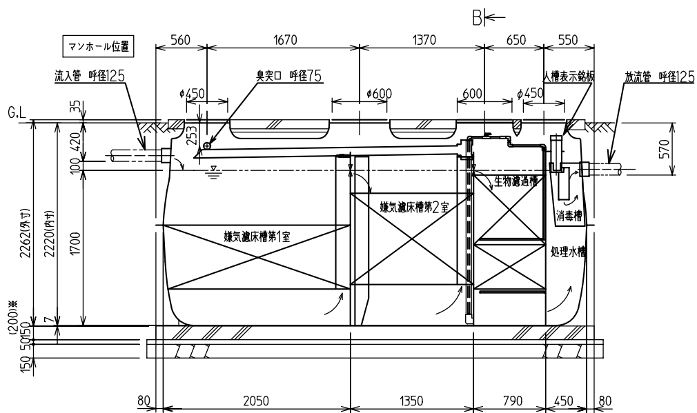
A-A'断面図
