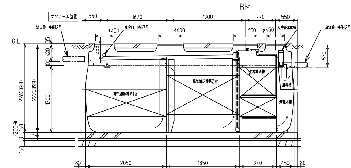
A-A'断面図
