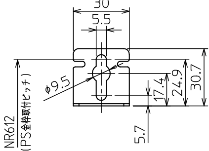
○C部詳細図(尺度1/2)
