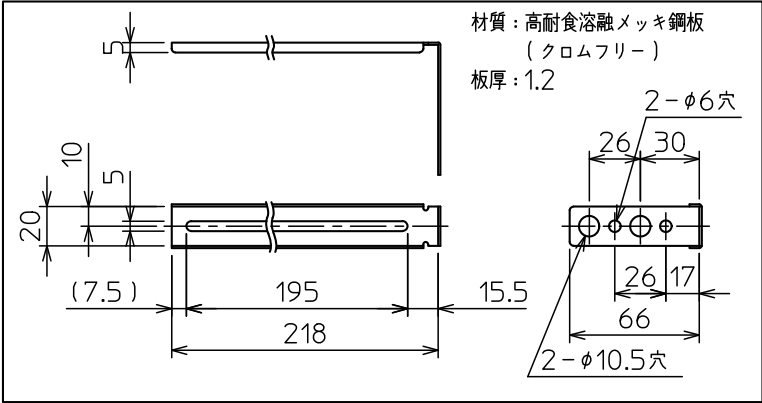
ロ本体取付板（付属部品）（尺度フリー）
