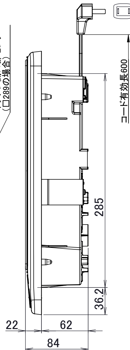
側面図
