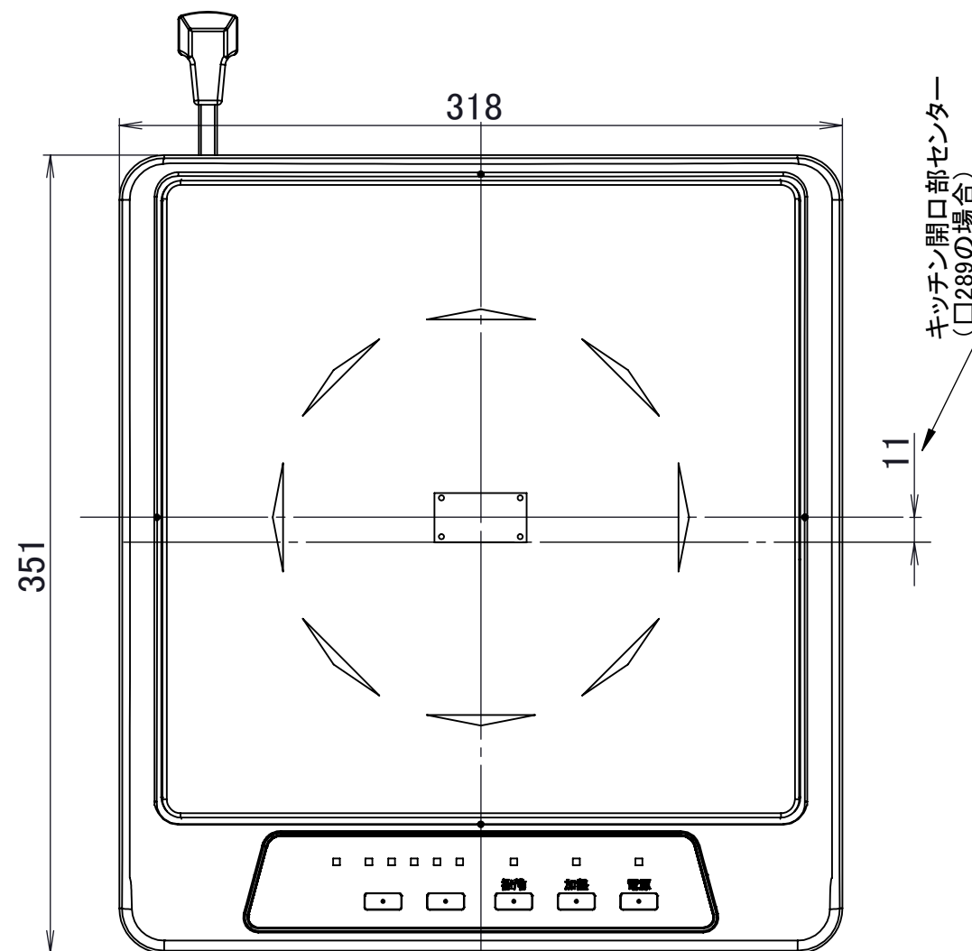
平面図
