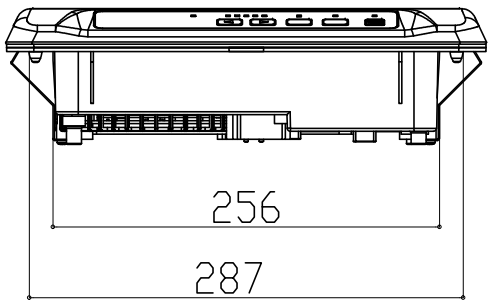
正面図
