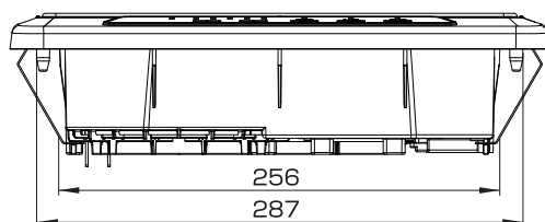
正面図
