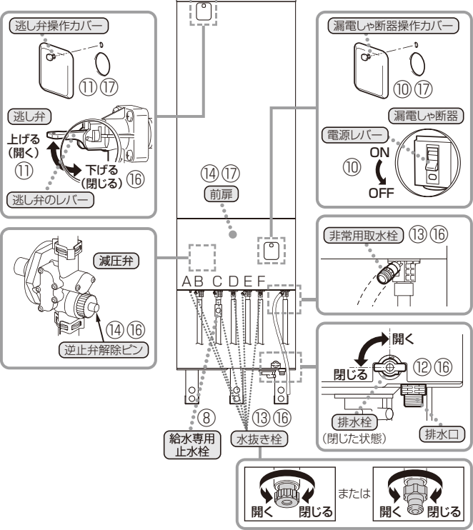
■貯湯ユニット
