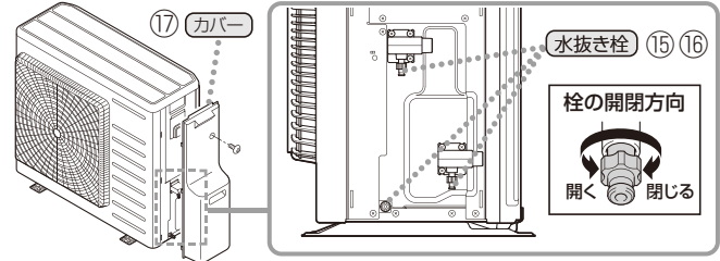
■ヒートポンプユニット
