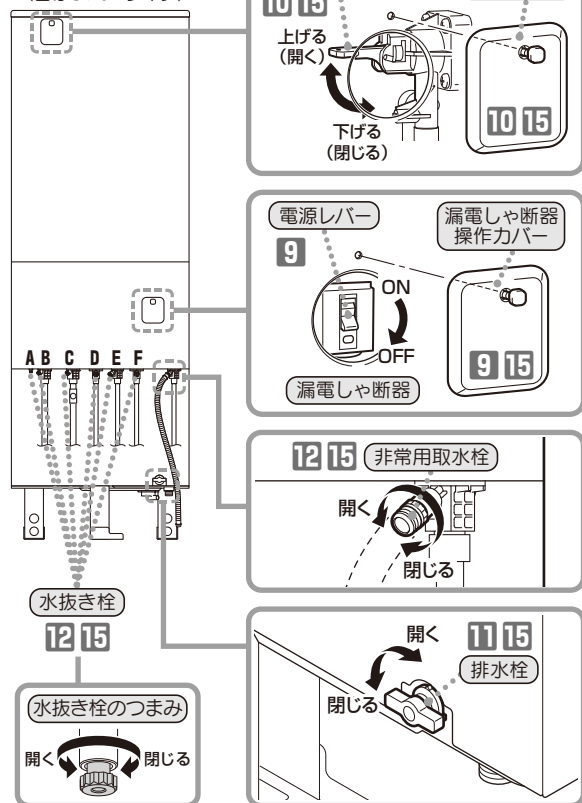
■貯湯ユニット (図は370Lタイプ)
