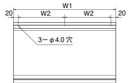
立面図
