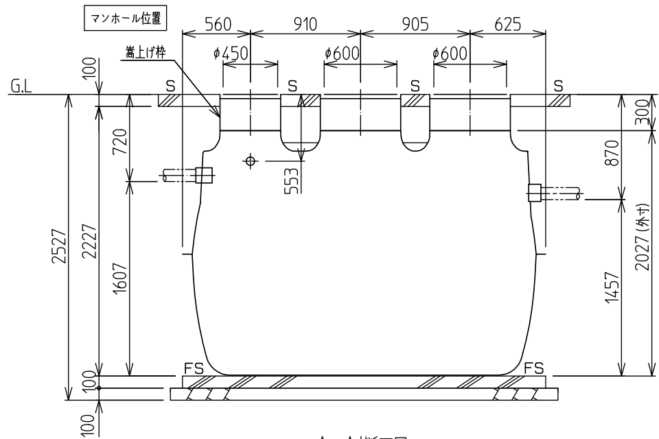
A-A'断面図
